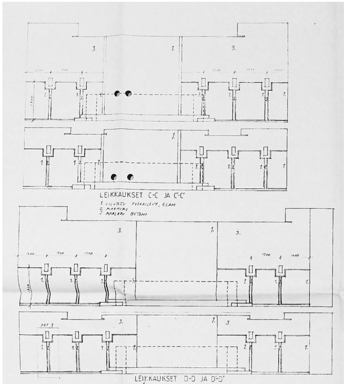
Istuntosalien seinäverhoukset ja detaljit. Seinäverhouksissa käytettiin pyökkiä, marmoria ja messinkilistoja. 1.3.1990, Arkkitehtuuritoimisto Kouvo & Partanen, SKA.
