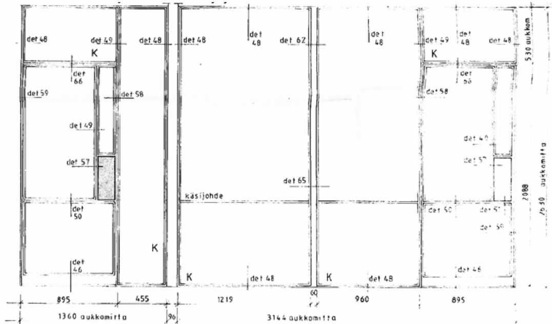
Ovikaavio ja lasiseinien teräsotet. 1.3.1990, Arkkitehtuuritoimisto Kouvo & Partanen, SKA.
