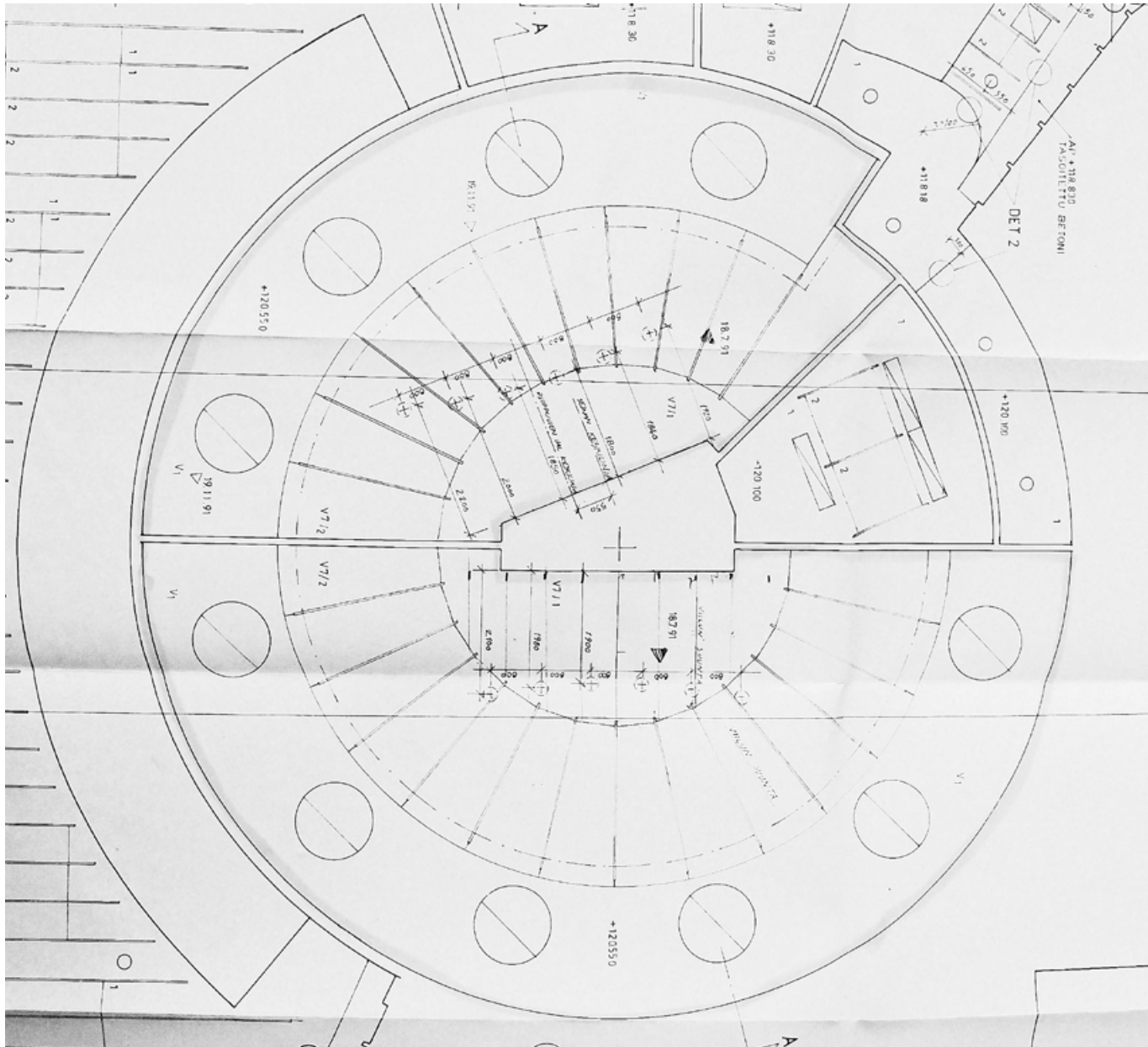
Alakattokuva istuntosalista, jossa esitetty kattoikkunat. Ote piirustuksesta. 19.11.1991, Arkkitehtuuritoimisto Kouvo & Partanen, SKA.
