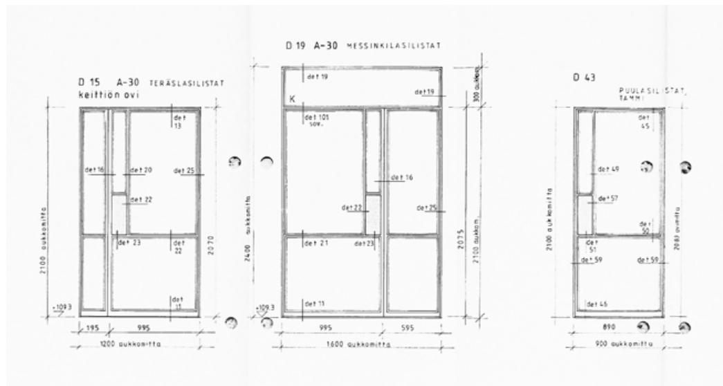
Teräslasiovia, 1.3.1990, Arkkitehtuuritoimisto Kouvo & Partanen, SKA.
