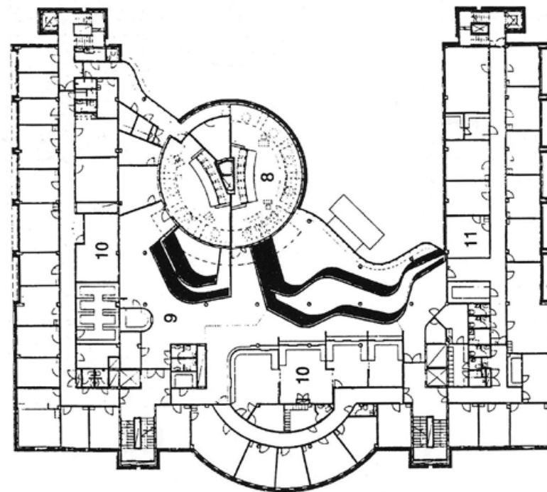
Kolmannen kerroksen pohjapiirustus. Arkkitehtuuritoimisto Kouvo & Partanen, Kuopion oikeus- ja poliisitalo esite, Rakennushallitus 1993.
