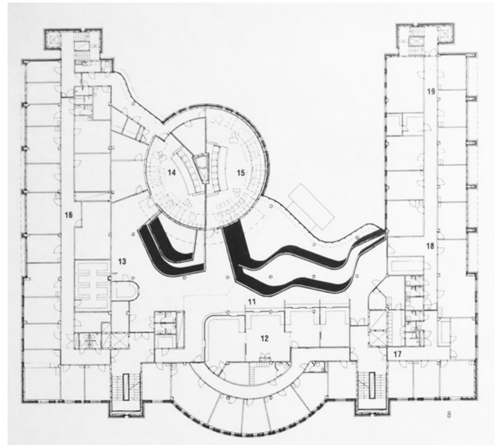
Arkkitehti-lehdessä 1993 esitetyt 2. kerroksen pohjapiirustukset. Arkkitehtuuritoimisto Kouvo & Partanen, Arkkitehti-lehti, 1/1993.
