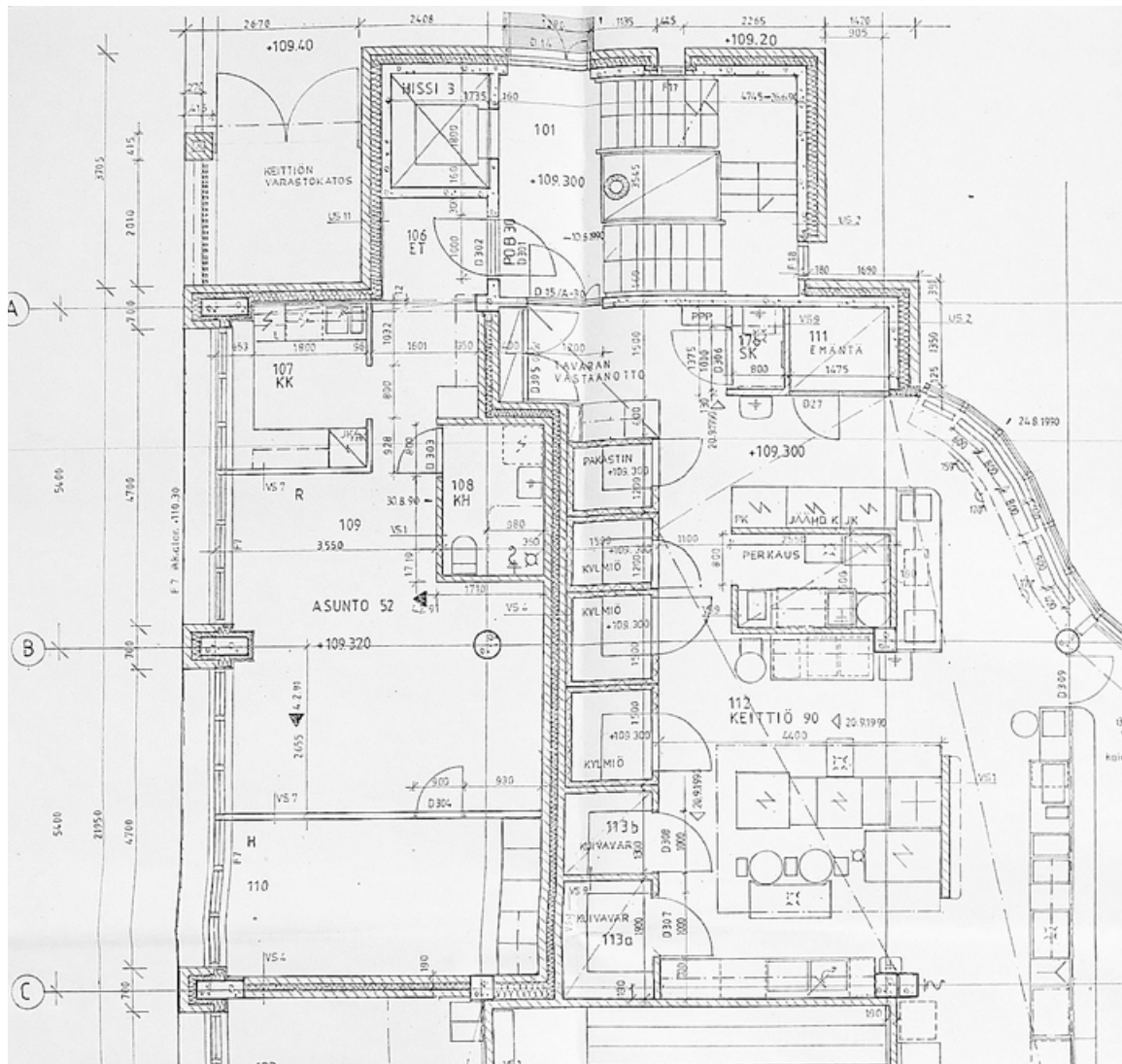
Rakennuksen eteläsiivessä oli alun perin talonmiehen asunto, joka on sittemmin muutettu toimistohuoneiksi. Arkkitehtuuritoimisto Kouvo & Partanen, 4.2.1991. SKA.
