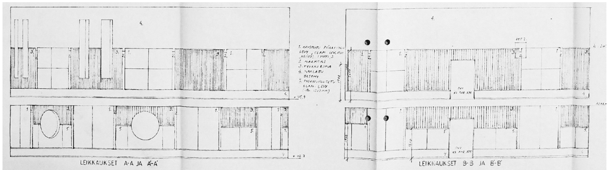
Istuntosalien seinäverhoukset ja detaljit. Seinäverhouksissa käytettiin pyökkiä, marmoria ja messinkilistoja. 1.3.1990, Arkkitehtuuritoimisto Kouvo & Partanen, SKA.
