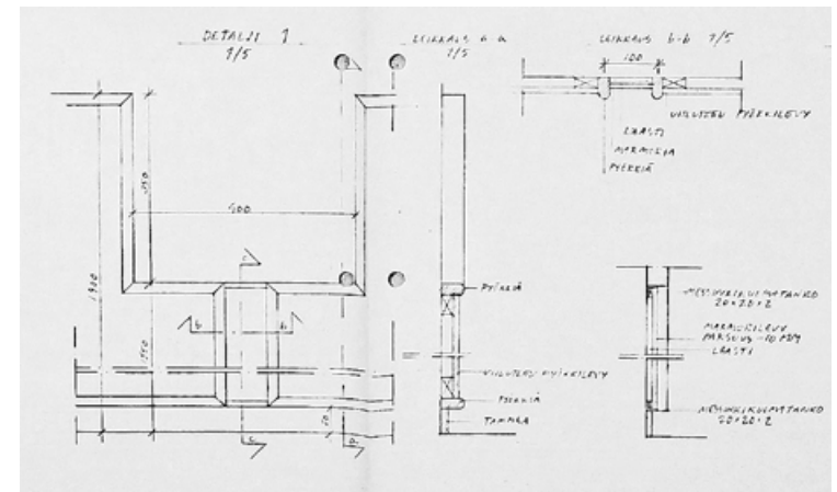
Istuntosalien seinäverhoukset ja detaljit. Seinäverhouksissa käytettiin pyökkiä, marmoria ja messinkilistoja. 1.3.1990, Arkkitehtuuritoimisto Kouvo & Partanen, SKA.
