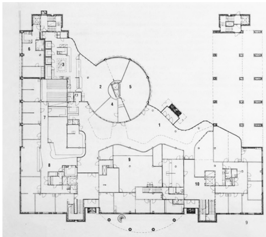
Arkkitehti-lehdessä 1993 esitetyt 1. kerroksen pohjapiirustukset. Arkkitehtuuritoimisto Kouvo & Partanen, Arkkitehti-lehti, 1/1993.
