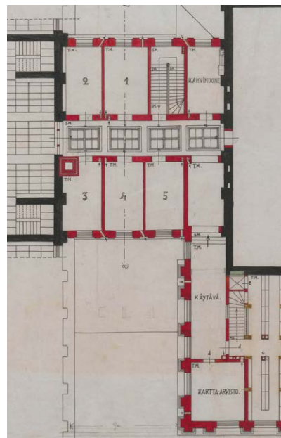
Kranckin päivämätön muutossuunnitelma, oletettavasti 1927. KA, Rakh II, Ibb.
