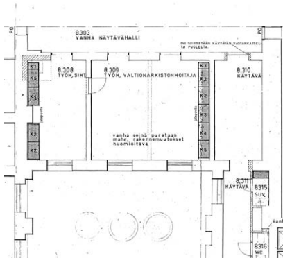
Alla Hanssonin pohja 1:50, 5.8.1968, ARK2017. SEN.
