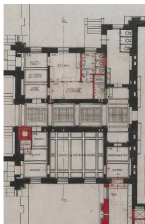
Päiväämätön suunnitelma, noin 1927, E. A. Kranck.
