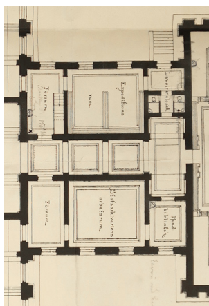
Pohjapiirustus 1885, Gustaf Nyström. KA1, Hea6, KA.
