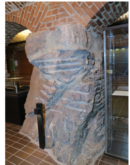
Näyttelytilan pilareista näkyy, että kellaritilaa on syvennetty. Vaakasuuntaiset kallioporausjäljet ovat peräisin Hanssonin vaiheesta, vähäiset pystysuuntaiset porareitit Nyströmin alkuperäistä kalliotyöstöä.
