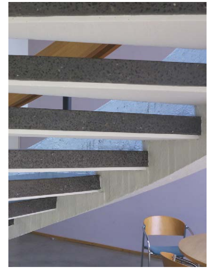
Portaan rakenteet paikalla valettua lautamuottipin- taista betonia, askellankut mosaikkibetonielement- tejä. Hanssonin suunnitelman mukaan betonipinto- jen tuli olla harmaita (naturel), mutta ne kuitenkin peittomaalattiin valkoisiksi.
