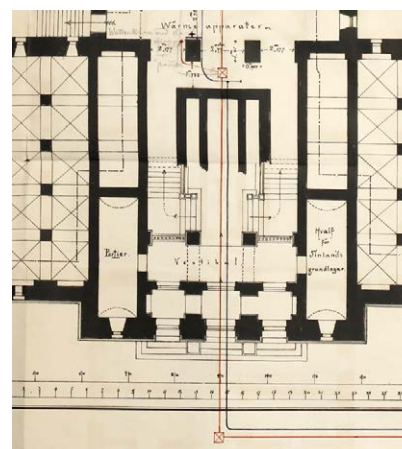
Pohjakerroksen pohjapiirustus 1885 toukokuulta. KA1, Hea6, KA.
