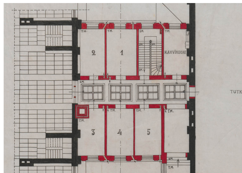
Kranckin päivämätön muutossuunnitelma, oletettavasti 1927. KA, Rakh II, lbb.
