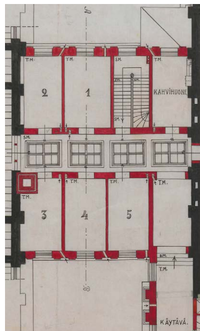
Vasemmalla Kranckin päiväämätön muutossuunnitelma, oletettavasti 1927. KA, Rakh II, lbb.
