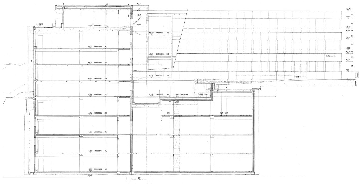
Leikkaus F-F, Ola Hansson 20.5.1968, pääpiirustussarja. SENA.
