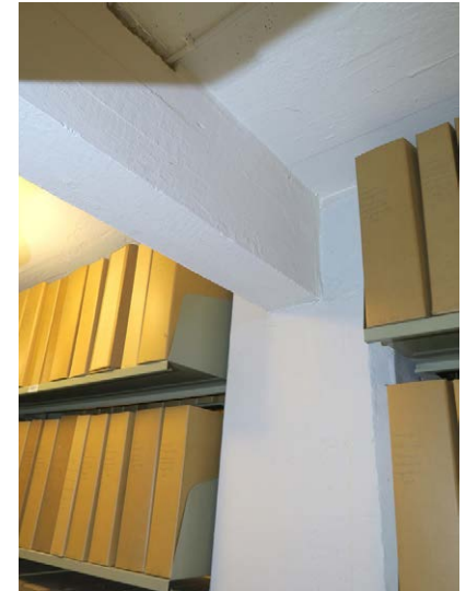
Makasiinin alkuperäiset rautarakenteet on valettu betoniin.
