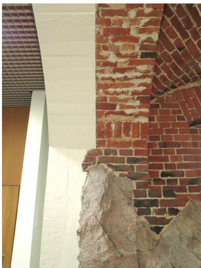
Kellarikerroksen rakennesauma uuden, betonista valetun keskushallin ja vanhan tiilestä muuratun virkailijakäytävän kohdalla.
