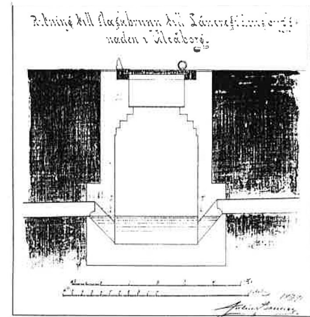
Kuva 52. Läänihallituksen liikakaivo, J.Basilier 1891
