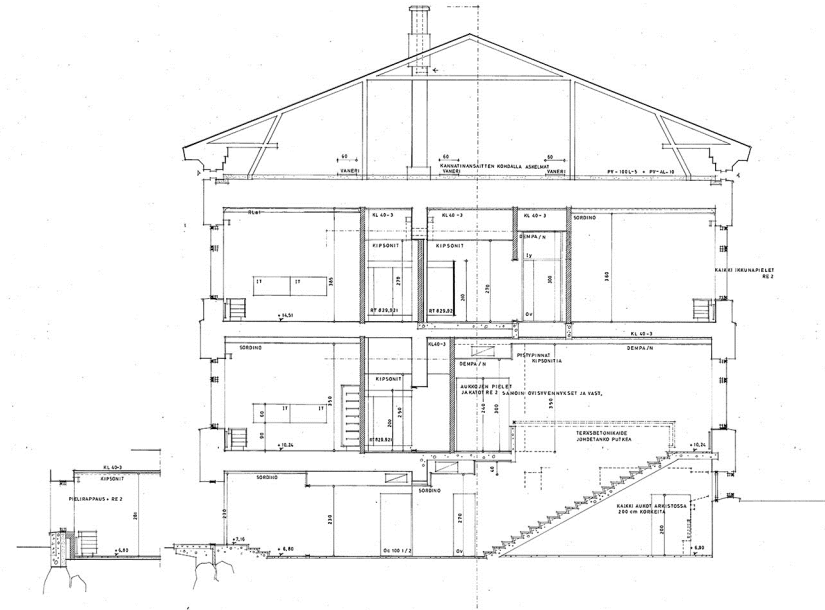
Kuva 63. Päärakennuksen leikkauspiirustus, uudet sisäportaat, Mikko Huhtela 1971.
