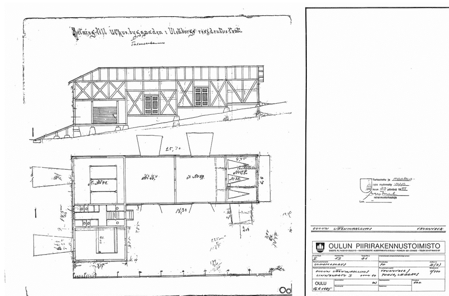
Kuva 186. Piharakennus, pohjapiirustus ja leikkaus, alkuperäispiirustuksen yhteyteen laadittu värisuunnitelma 1985.
