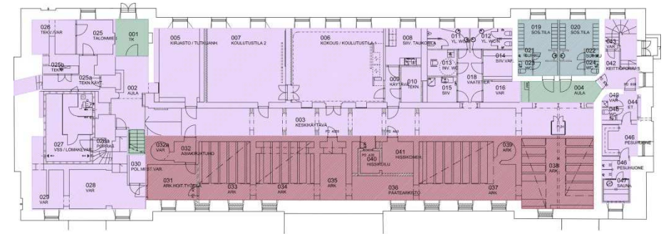
KELLARIKERROS
