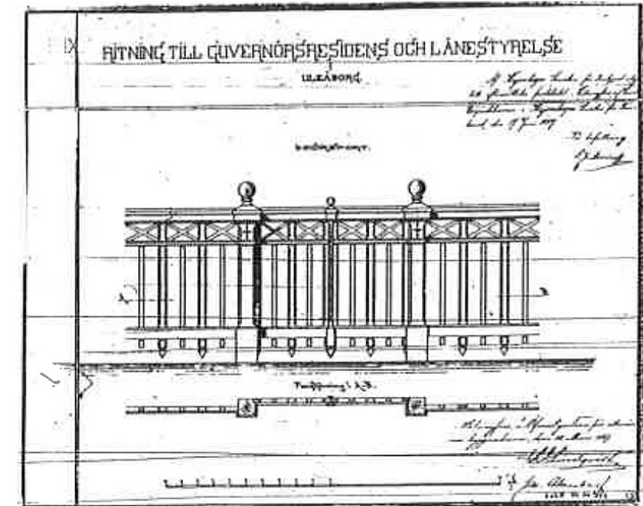
Kuva 34. Tonttiaidan piirustus.
