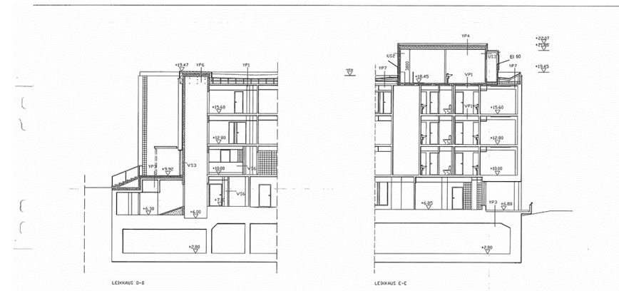
Kuva 155. Leikkauspiirustukset uuden hissin rakentamiseksi.
