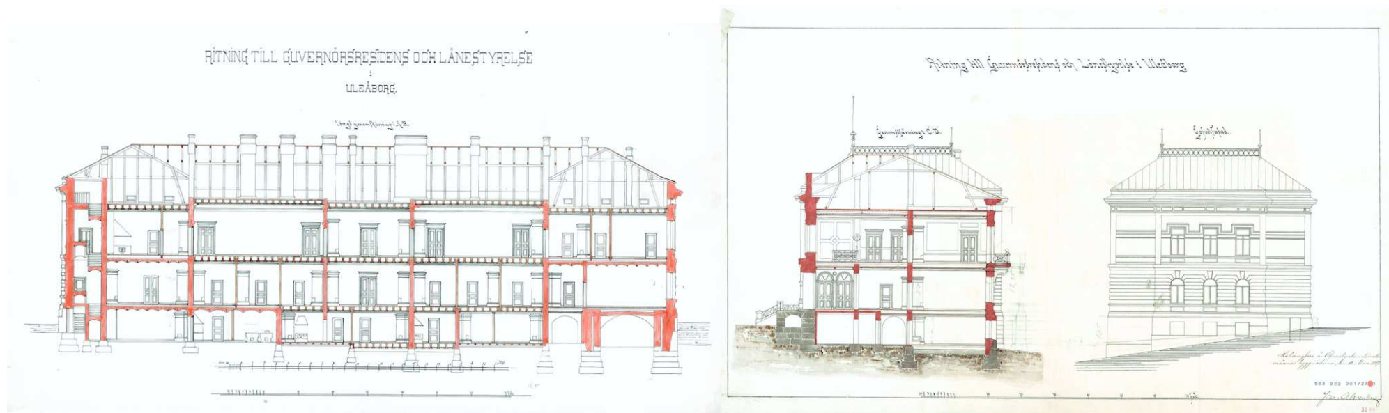
Kuva 32. Lopullisen hyväksytyn suunnitelman leikkaukset ja päätyjulkisivu
