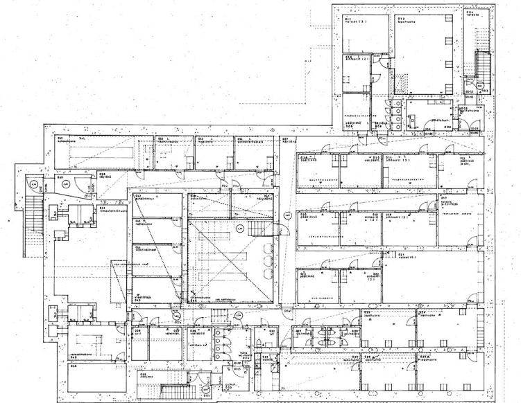
Kuva 138. Kellarikerroksen pohjapiirustus 1969.
