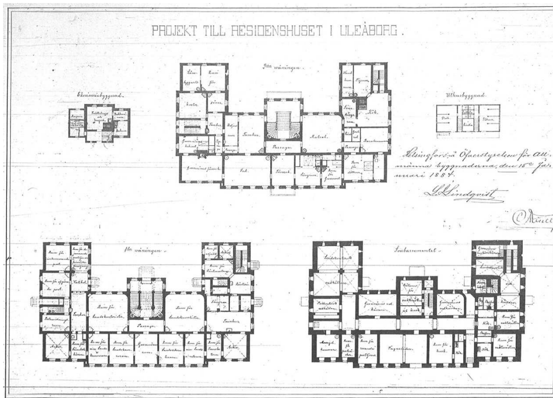
Kuva 19. Kiseleffin luonnokset. Maaherran työhuone on sijoitettu keskeisesti sisäänkäyntiä vastapäätä siten, että ikkunat avautuvat puistoon. Läpikuljettavat lääninkonttorin ja -kanslian konttoristien salit on sijoitettu kadun puolelle ja korkeampien virkamiesten erilliset huoneet puiston puolelle. Käsiarkisto, lääninkassa, sivuportait ym. tilat on sijoitettu rakennuksen sivusiipiin. Sisäänkäynnit on osoitettu myös päädyistä, joista pääsee erillisiin postinkäsittelyhuoneisiin ja lääninkassaan. Edelleen erillinen sisäänkäynti on kuulusteluihin tulevia tai kuljetuksiin passitettavia vankeja varten. Herran huoneistoon yläkerrassa kuuluu maaherran kabinetti etuhuoneineen sekä poikien ja palvelijan huoneet. Näille huoneille on erillinen sisäänkäynti ja porrashuone. Rouvan huoneiston muodostaa rouvanhuone, lastenkamari ja sänkykamari. Näihin tiloihin liittyvät myös ruokasali, keittiö, palvelijainhuone ja muut taloustilat. Keittiölle on oma porras.
