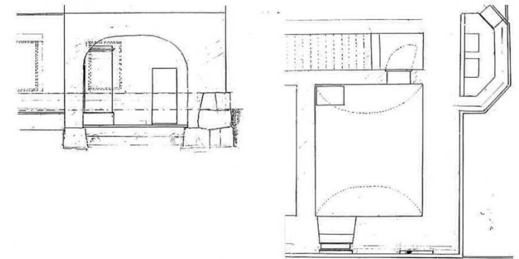
Kuva 43. Sunnitelma Franzenin talon nurkkahuoneen holvaamiseksi lääninkassan tarpeisiin, J. Basilier 1886
