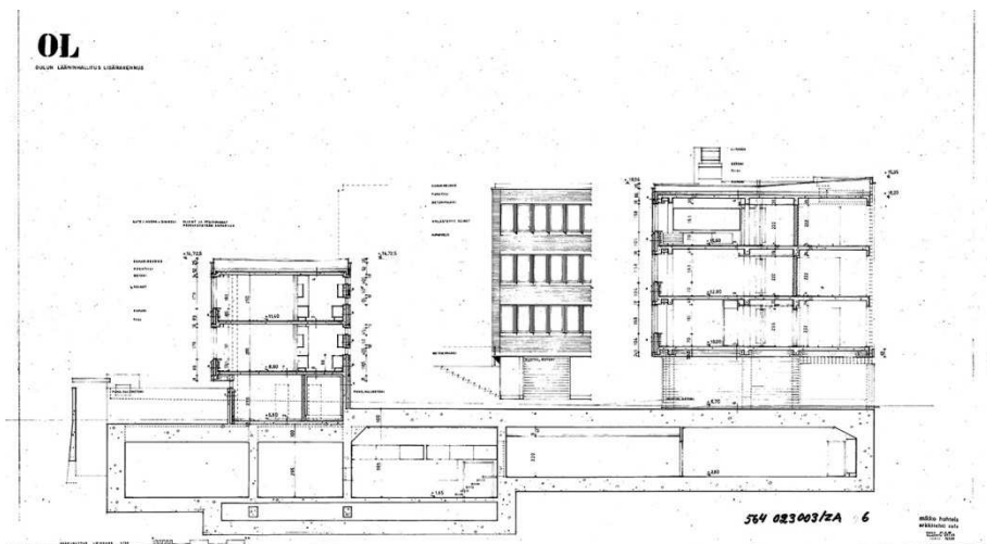
Kuva 139. Leikkauspiirustus 1969.
