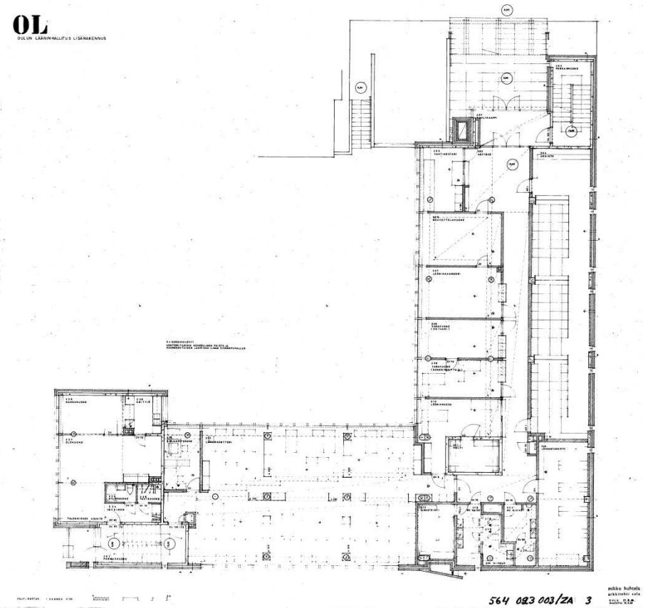
Kuva 141. Pohjapiirustus, 1. kerros 1969.
