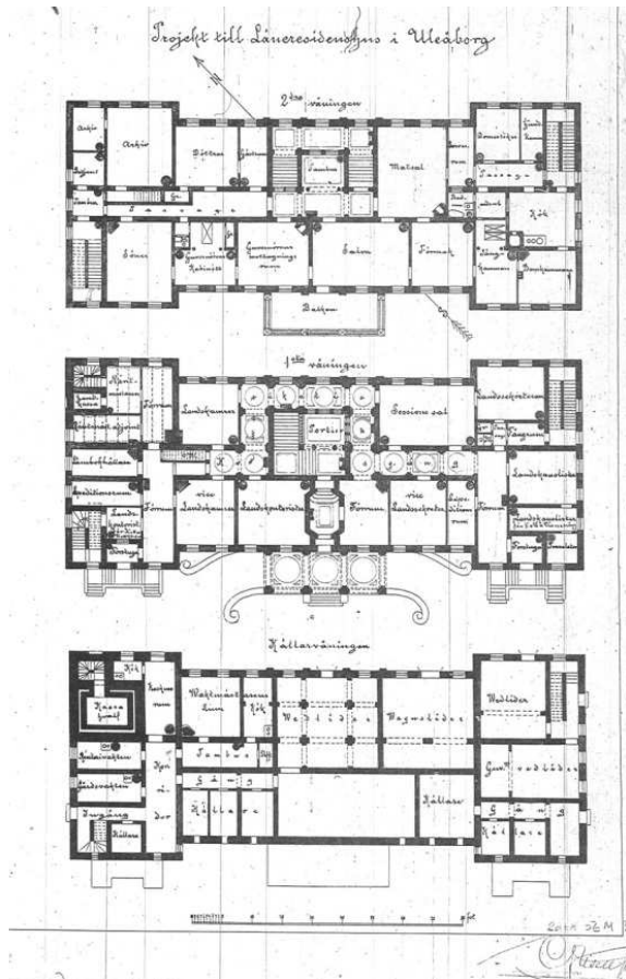
Kuva 28. Myöhempiä Kiseleffin pohjaluonnoksia.
