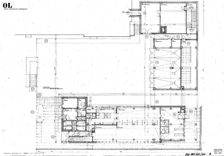
Kuva 140. Pohjapiirustus, pohjakerros 1969.
