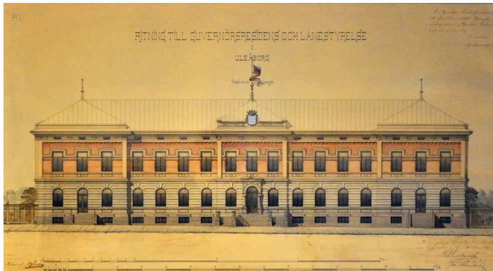
Kuva 31. Lopullisen hyväksytyn suunnitelman julkisivut
