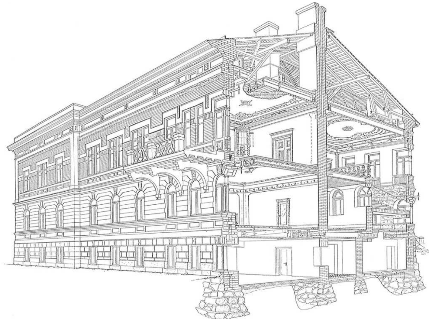
Kuva 101. Leikkausperspektiivi (Weikko Kotila 1994).
