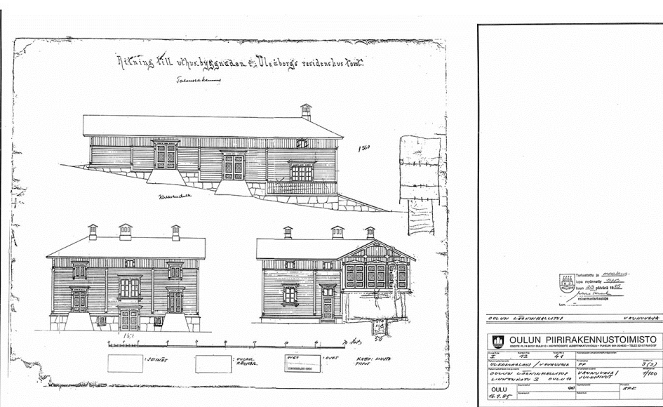
Kuva 187. Piharakennus, julkisivut, alkuperäispiirustuksen yhteyteen laadittu värisuunnitelma 1985.
