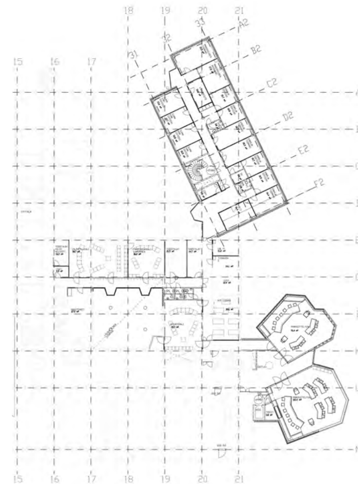
kuva 5.53 Oikeustalon K-, T- ja I-osien laajennukset 3. krs pohjapiirustuksessa. Samassa muotokuvassa näkyvät entisen arkiston tilalle rakennetut pienemmät istuntosalit. Piirustus Arkkitehdit Leppänen Oy, Senaatin arkisto
