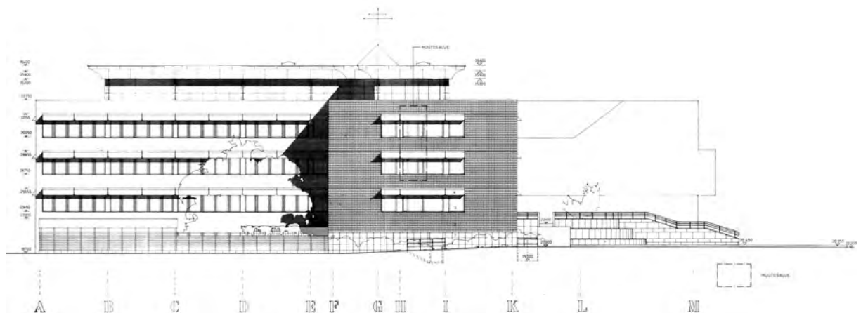
kuva 5.24 Julkisivu pohjoiseen Valkoisenlähteentielle. Piirustus Arkkitehtitoimisto Kaarlo Leppänen Oy, Senaatin arkisto
