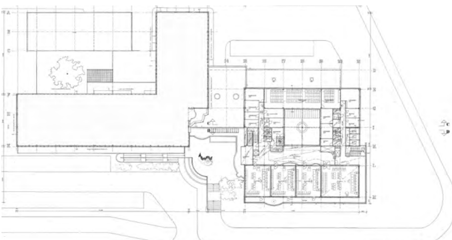
kuva 5.7 Ensimmäisen rakennusvaiheen 3. kerroksen pohjapiirustus. Piirustus Arkkitehtitoimisto Kaarlo Leppänen Oy, Senaatin arkisto
