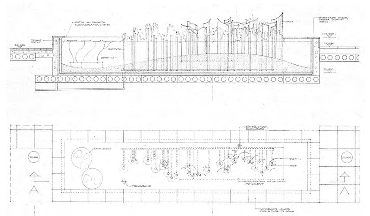
kuva 5.16 Pääsisääkäyntitasanteelle suunniteltu suihkulähde. Piirustus Arkkitehtitoimisto Kaarlo Leppänen Oy, Senaatin arkisto
