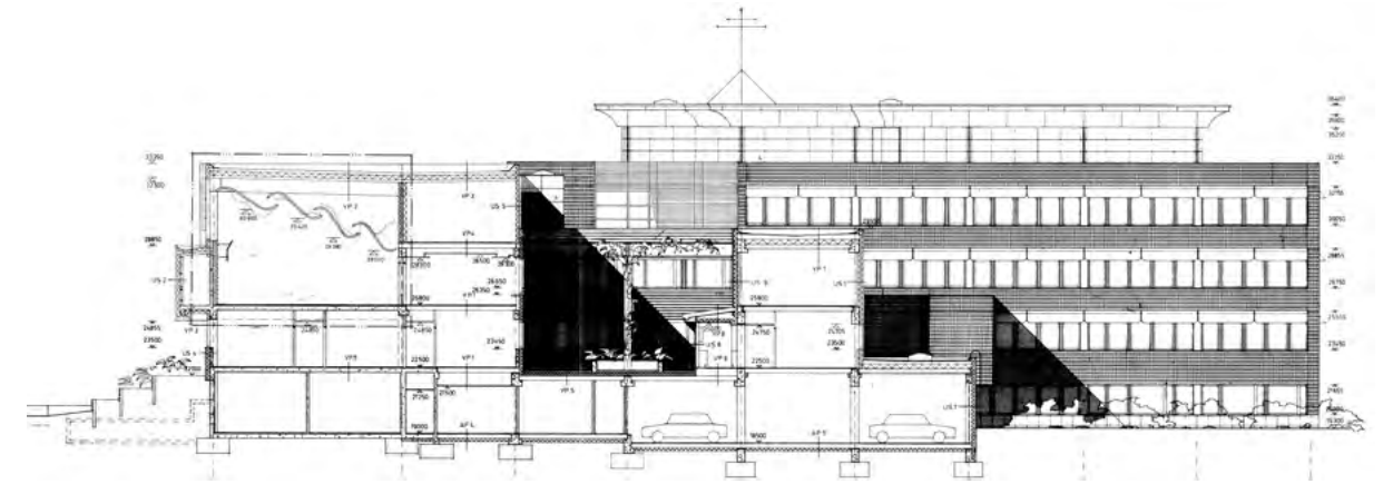
kuva 5.332 Leikkauspiirustus, jossa näkyy atriumpihan alkuperäinen suunnitelma. Piirustus Arkkitehti-toimisto Kaarlo Leppänen Oy, Senaatin arkisto
