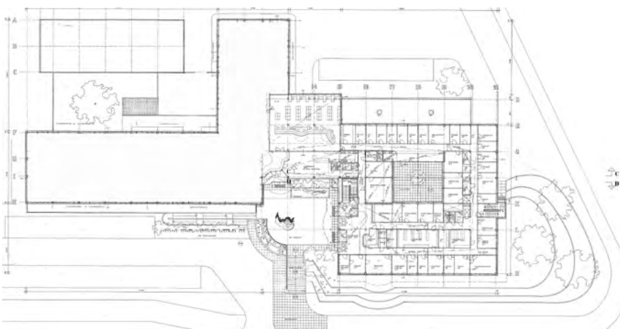
kuva 5.6 Ensimmäisen rakennusvaiheen 2. kerroksen pohjapiirustus. Piirustus Arkkitehtitoimisto Kaarlo Leppänen Oy, Senaatin arkisto
