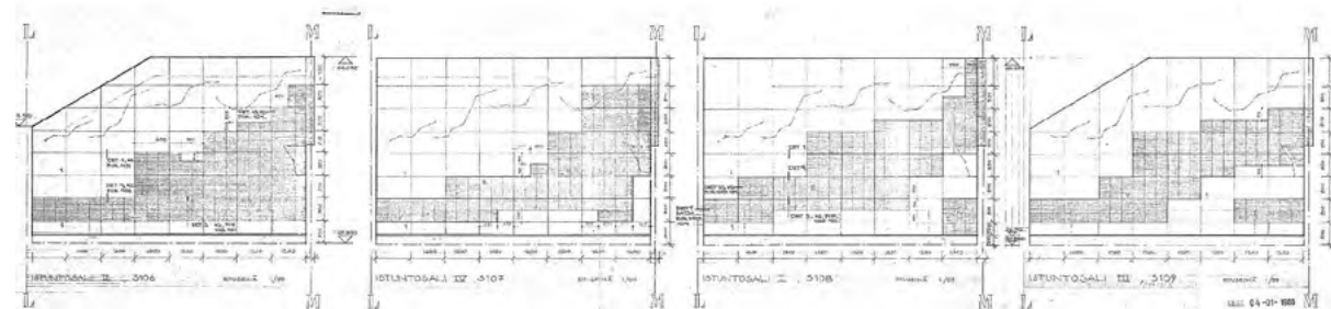
kuva 5.311 Vanhojen istuntosalien seinäkaavioissa on akustiikkapintojen suunnitelma. Alakaton akustoivat elementit olivat suunnitelmissa ensin vapaamuotoisempia, lopullinen toteutus oli säännönmukaisena toistuva siiveke. Piirustus Arkkitehtitoimisto Kaarlo Leppänen Oy, Senaatin arkisto
