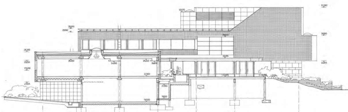
kuva 5.19 Leikkaus sisäänkäyntitasanteen kohdalta kohti oikeustaloa. Piirustus Arkkitehtitoimisto Kaarlo Leppänen Oy, Senaatin arkisto
