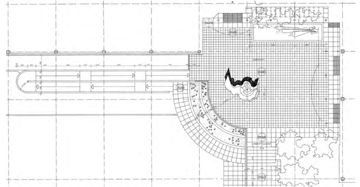
kuva 5.15 Pääsisääkäynnin suunnitelma, jossa näkyy detaljien painottuminen tärkeään osaan rakennusta. Sisääkäyntitasolle on suunniteltu suihkulähde ja veistos. Veistos sijoitettiin myöhemmin Kielotien varteen eikä tässä suunniteltuun kohtaan. Piirustus Arkkitehtitoimisto Kaarlo Leppänen Oy, Senaatin arkisto
