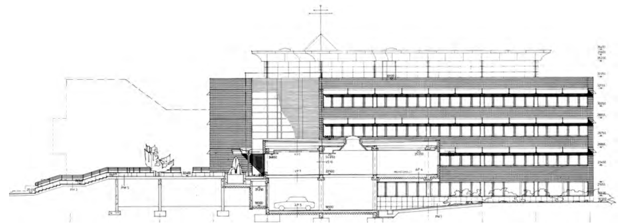
kuva 5.33 Leikkaus sisääntuloon kohdalta. Piirustus Arkkitehtitoimisto Kaarlo Leppänen Oy, Senaatin arkisto
