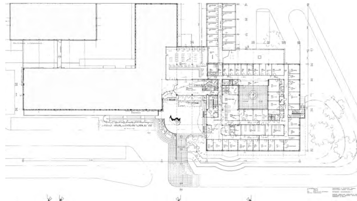
kuva 5.57 Vuonna 1995 valmistuneen laajennuksen pohjapiirros. Piirustus Arkkitehtitoimisto Kaarlo Leppänen Oy, Senaatin arkisto
