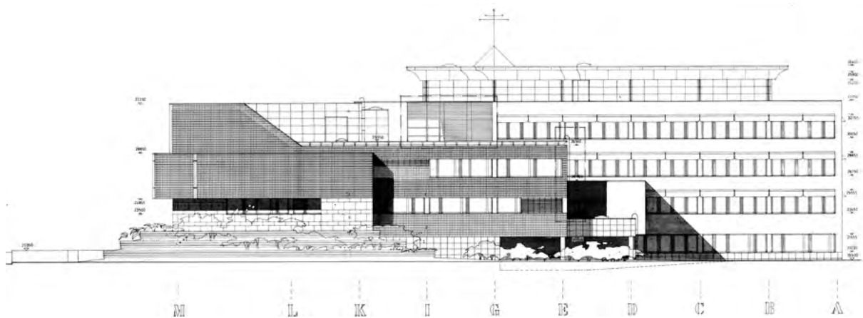
kuva 5.22 Julkisivu etelään Esikkotielle. Piirustus Arkkitehtitoimisto Kaarlo Leppänen Oy, Senaatin arkisto
