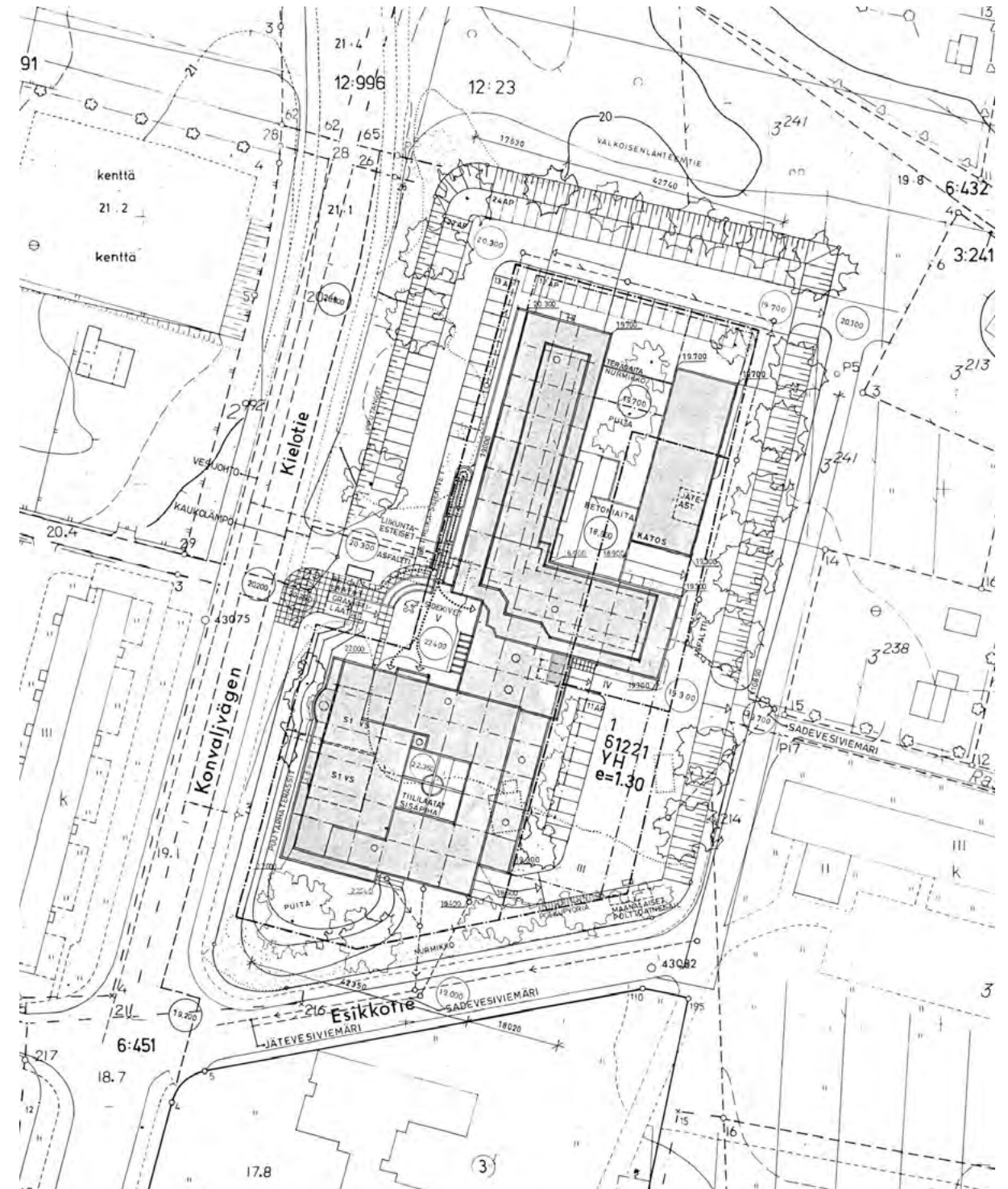
kuva 5.11 Ensimmäisen rakennusvaiheen asemapiirros vuodelta 1986. Poliisitalon osa on L-muotoinen, oikeustalo neliö, jonka keskellä on atriumpiha. Rakennuksia yhdistää nivelosa. Pääsisäänkäyntien tasanne on nivelosan edustalla. Poliisitalon pihassa on katos, joka korvattiin muutaman vuoden päästä saman muotoisella laajennusosalla. Piirustus kiinteistön arkistosta, Arkkitehtitoimisto Kaarlo Leppänen Oy
