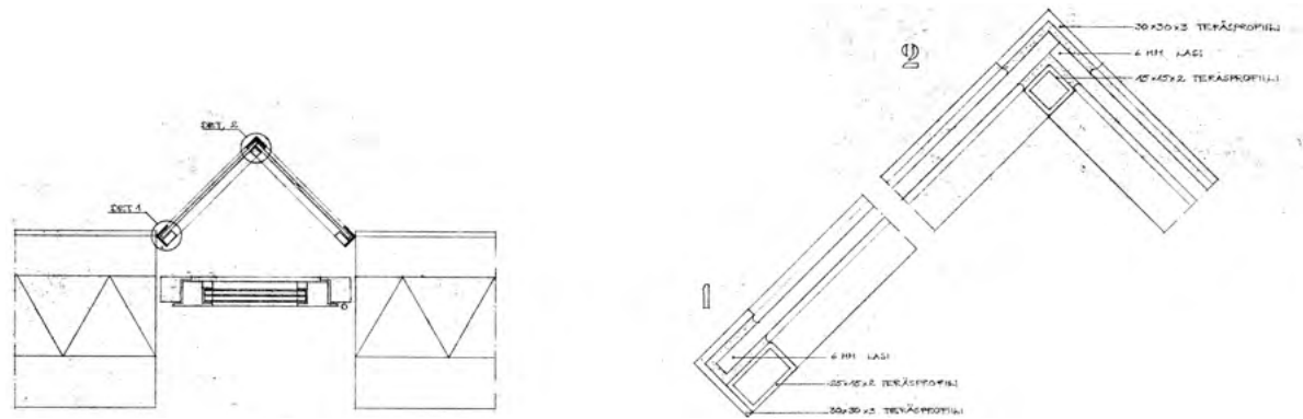
kuva 5.25 Kielotien julkisivun prisman muotoinen ikkuna, joka tarjoaa kurkistusaukon oikeussalien takakäytävästä ulos. Piirustus Arkkitehtitoimisto Kaarlo Leppänen Oy, kiinteistön arkisto
