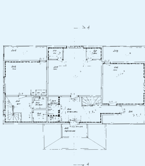
POHJAPIIRROS, ULLAKKO
