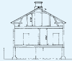
Leikkaus A-A
