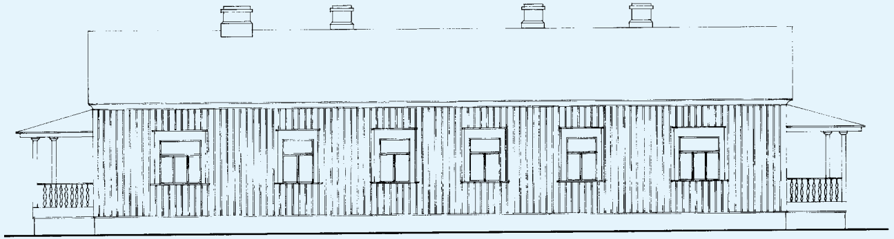
SIVU LOUNAASEEN
