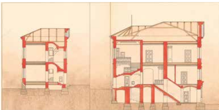
Ahrenbergin 27.6.1913 allekirjoittamat leikkauspiirustukset. Vasemalla pihasiiven, oikealla runkorakennuksen leikkaus. Kansallisarkisto.
