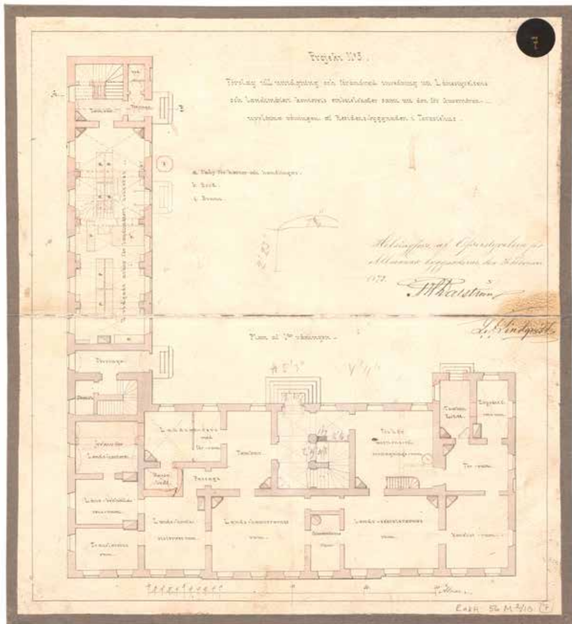
Dahlströmin 26.2.1872 allekirjoittama muutospiirustus. Pihasiiven laajennusosa on kuvattu punaisella. Ensimmäinen kerros, jonka maanmittauskonttorin käytössä ollutta arkistosalia laajennettiin. Samalla tehtiin väliseinä- ja tulisijamuutoksia myös vanhaan osaan. Kansallisarkisto.
