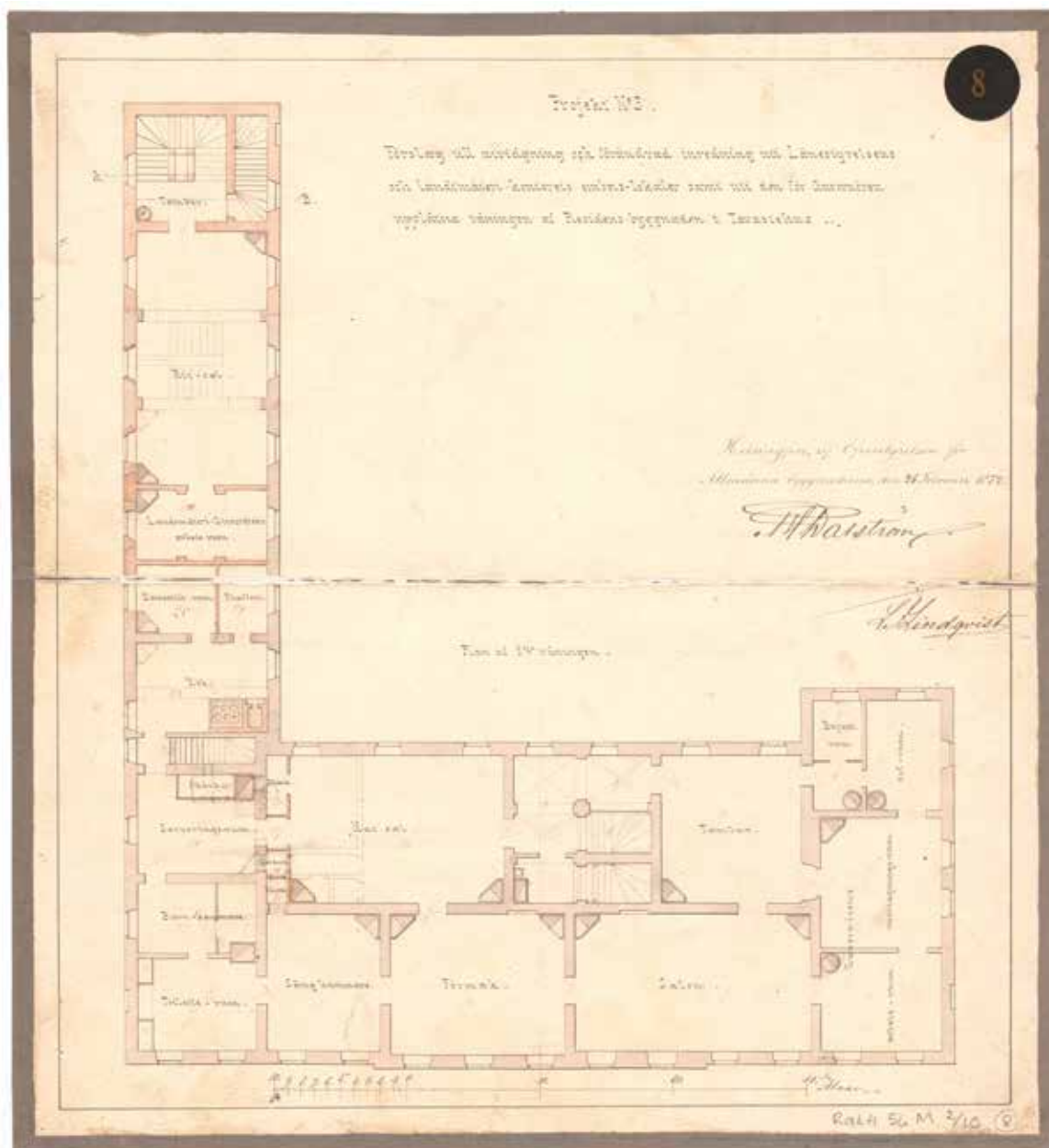
Dahlströmin 26.2.1872 allekirjoittama muutospiirustus. Pihasiiven laajennusosa on kuvattu punaisella. Toinen kerros, jossa tehtiin laajennuksen lisäksi sisätilamuutoksia koko pihasiivessä. Kansallisarkisto.
