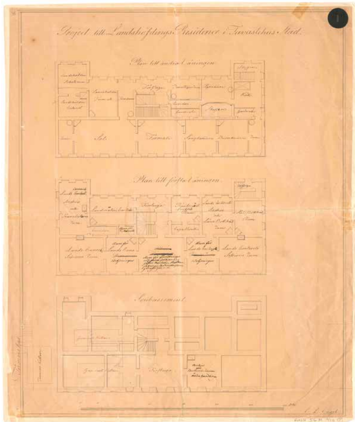
Engelin ensimmäinen suunnitelma lääninhallituksen talon kolmen kerroksen pohjapiirustuksiksi. Kansallisarkisto.
