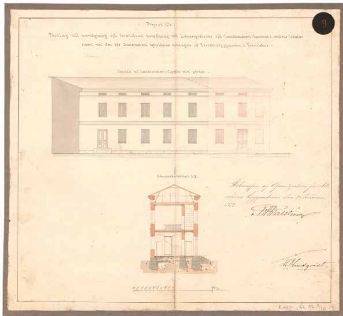
Dahlströmin 26.2.1872 allekirjoittama muutospiirustus. Lisäsiiven pihajulkisivu ja laajennusosan leikkaus. Kansallisarkisto.
