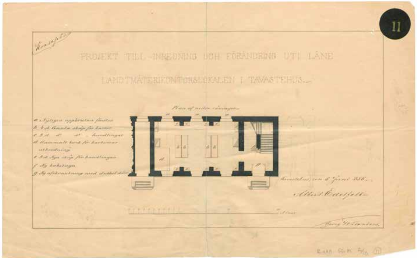
C. A. Edelfeltin 6.7.1856 allekirjoittama muutospiirustus. Ensimmäisen kerroksen pohjapiirustus. Kansallisarkisto.
