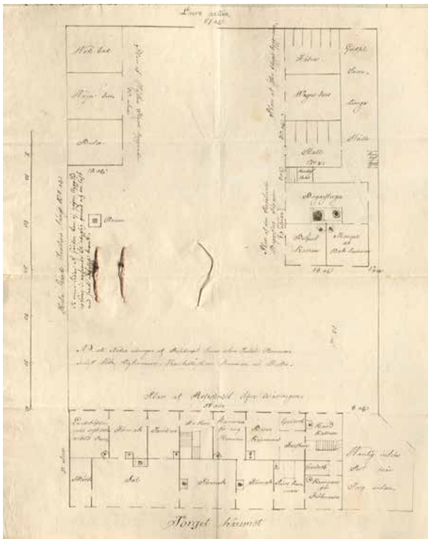
1700-luvun palaneen maaherran talon pihasta säilynyt kaavio liittyy lupahakemukseen piharakennuksen laajennusta koskien. Sommitelma on samankaltainen kuin Engelin asemapiirroksessa, joskin piharakennuksen muodostavat U-muodon sijaan kaksi erillistä rakennusta, joita yhdistää aita pohjoisessa.
