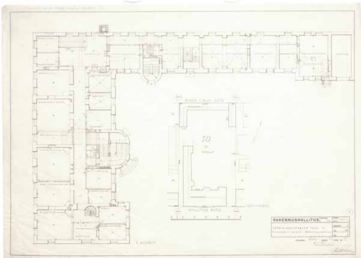
Muutospiirustukset on allekirjoittanut Väinö Vähäkallio 24.2.1938. Kuvassa ensimmäisen kerroksen pohjapiirros sekä asemapiirros. Kansallisarkisto.
