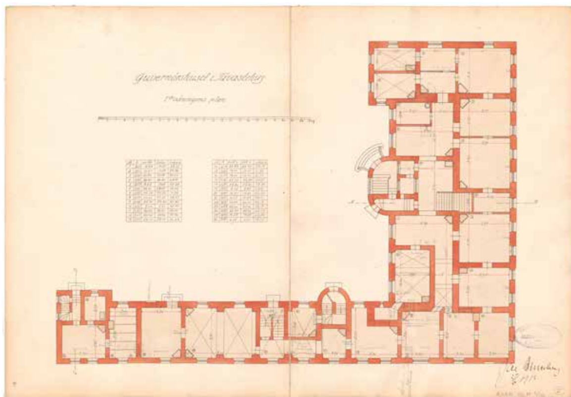
Ahrenbergin 27.6.1913 allekirjoittama ensimmäisen kerroksen pohjapiirustus. Kansallisarkisto.
