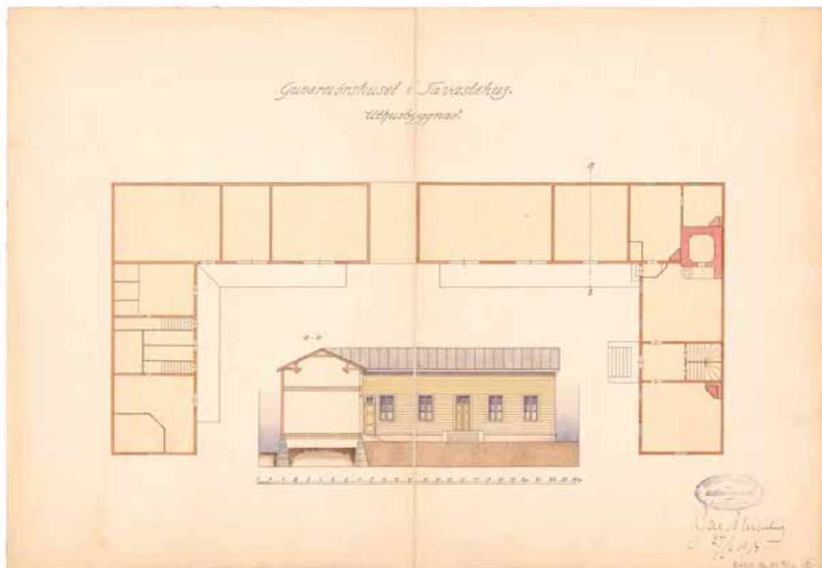
Ahrenbergin 27.6.1913 allekirjoittama piharakennuksen pohjapiirustus, leikkaus ja pihajulkisivu. Kansallisarkisto.
