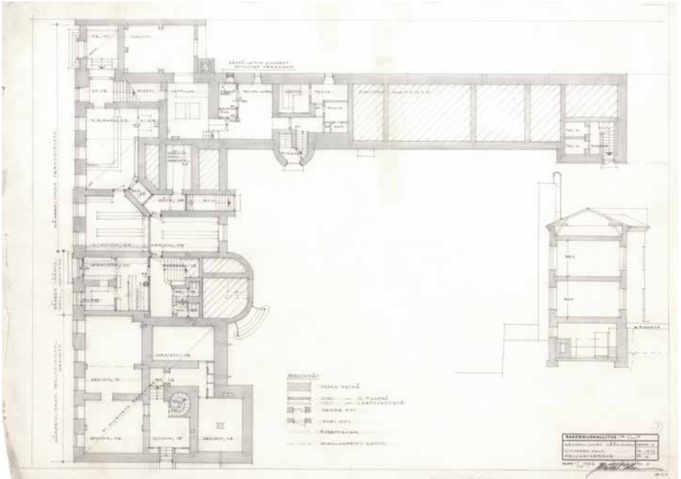
Muutospiirustukset on piirtänyt rakennushallituksessa J. Laurila ja ne on päivätty 1.10.1966. Kuvassa kellarin pohjapiirros sekä leikkaus. Kansallisarkisto.
