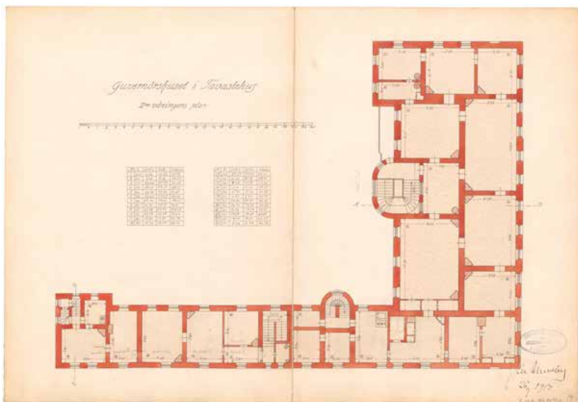
Ahrenbergin 27.6.1913 allekirjoittama toisen kerroksen pohjapiirustus. Kansallisarkisto.
