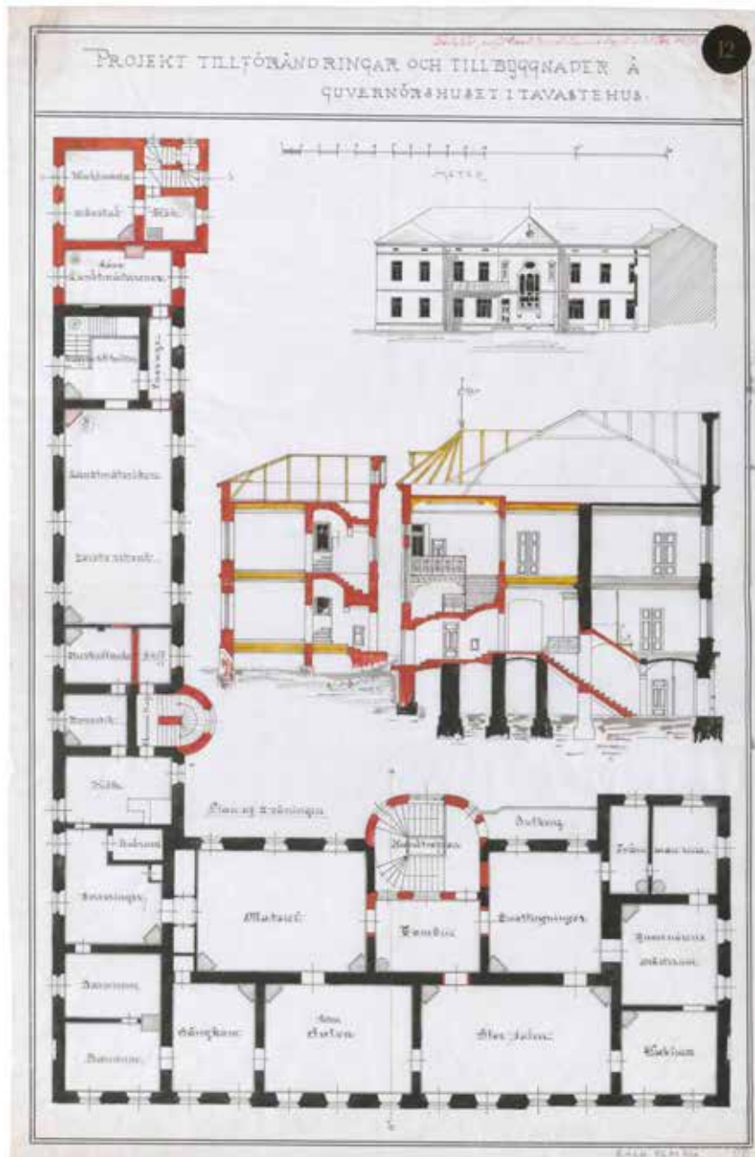
Caweenin muutospiirustus, runkorakennuksen pihajulkisivu, leikkaus ja toisen kerroksen pohjapiirustus. Kansallisarkisto.
