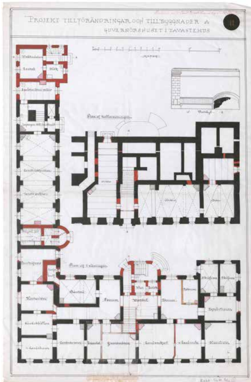
Caweenin muutospiirustus, kellarikerros ja ensimmäinen kerros. Rakennukseen toteutettiin kaksi uutta kaarevaa porrashuonetta ja pihasiipeä laajennettiin entisestään. Kansallisarkisto.
