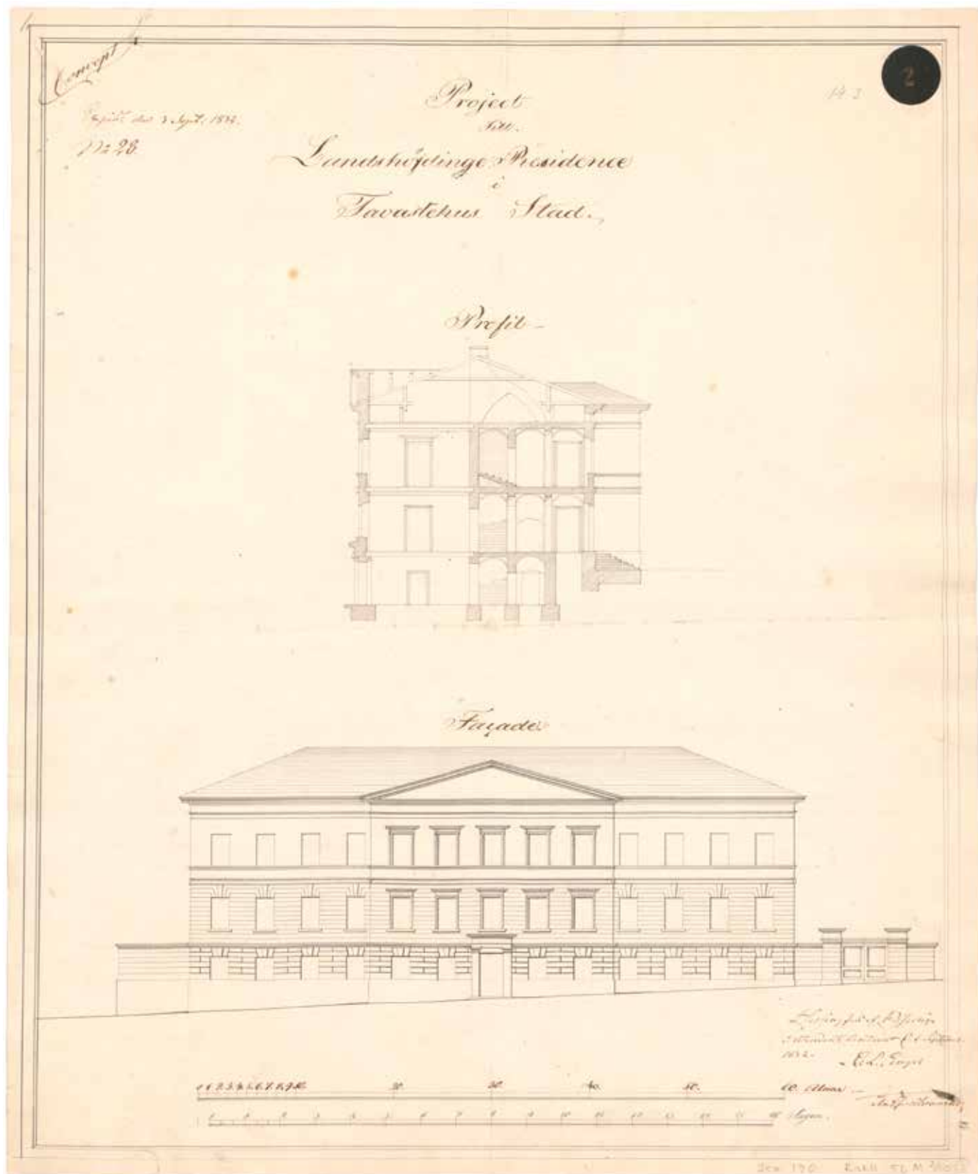
Leikkaus ja julkisivu. Engelin allekirjoittama piirustus on vuodelta 1832. Kansallisarkisto.
