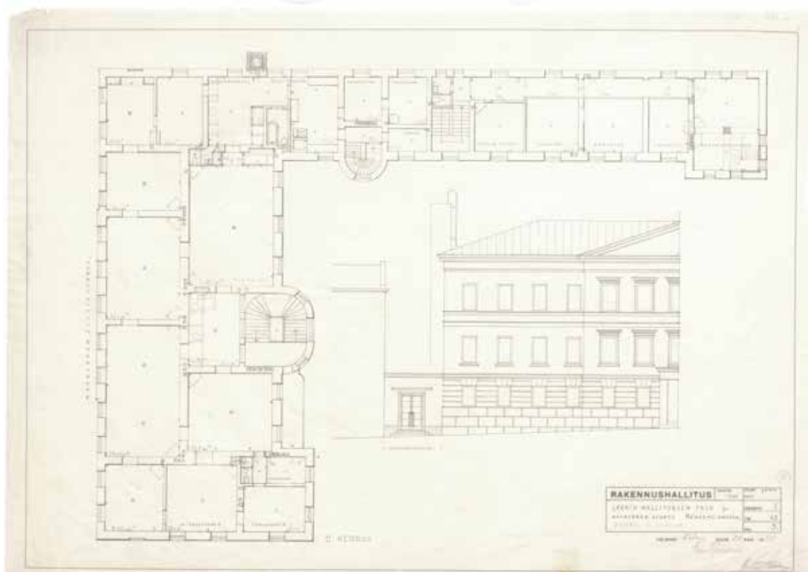
Muutospiirustukset on allekirjoittanut Väinö Vähäkallio 24.2.1938. Kuvassa toisen kerroksen pohjapiirros sekä julkisivuote. Kansallisarkisto.
