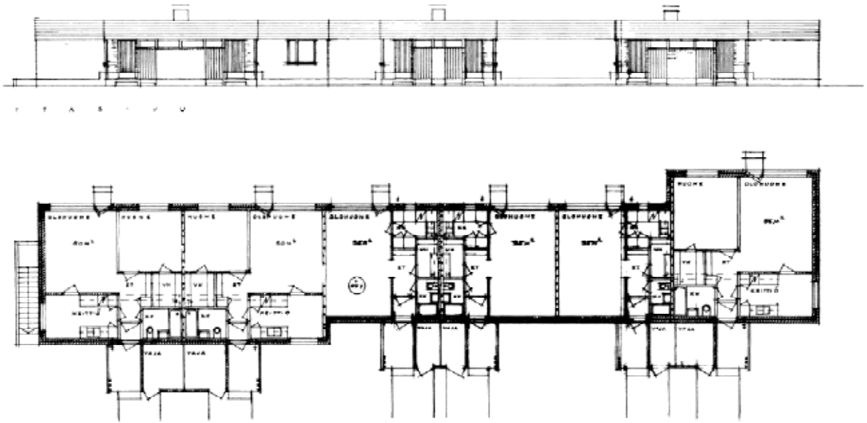
Henno Kamppurin julkisivu- ja pohjapiirustukset, jotka on päivätty 16.3.1970.
