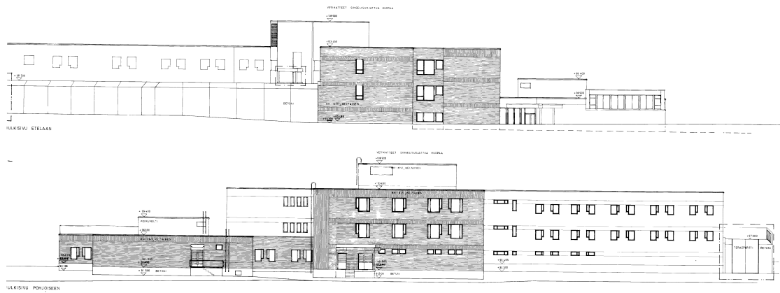
Vankisairaalan etelä- ja pohjoisjulkisivut. Veli Paatelan piirustus 11.9.1985
