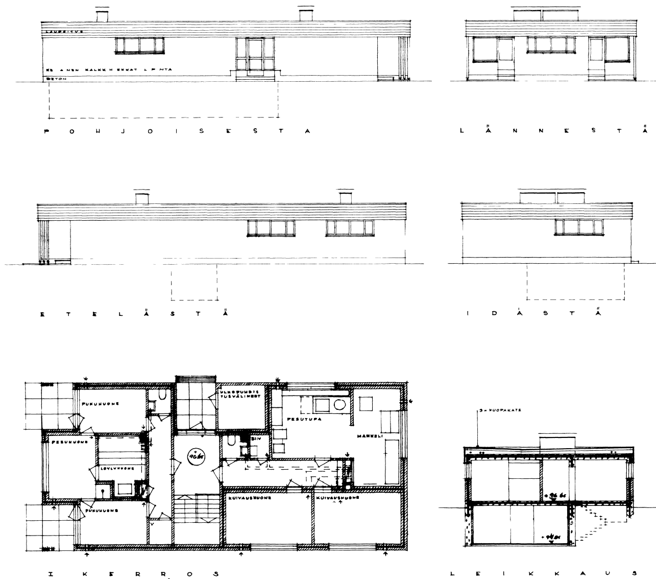
Henno Kamppurin julkisivu-, pohja- ja leikkauspiirustukset vuodelta 1970. Senaatti-kiinteistöt.
