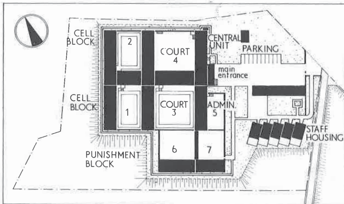
Aschaffenburgin vankilan asemapiirros ja valokuvia teoksessa Prison Architecture (Di Gennaro 1975, 121).
