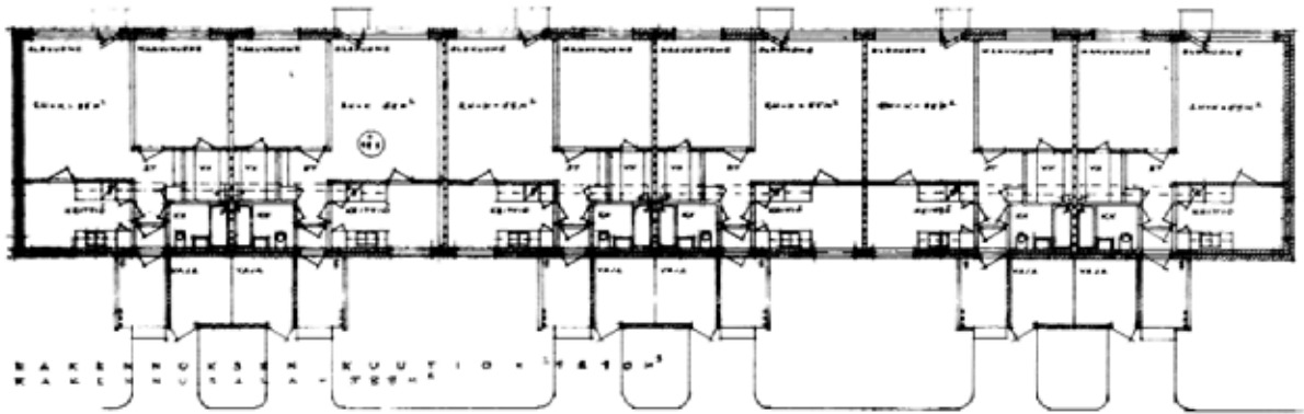
Henno Kamppurin julkisivu- ja pohjapiirustukset, jotka on päivätty 16.3.1970.
