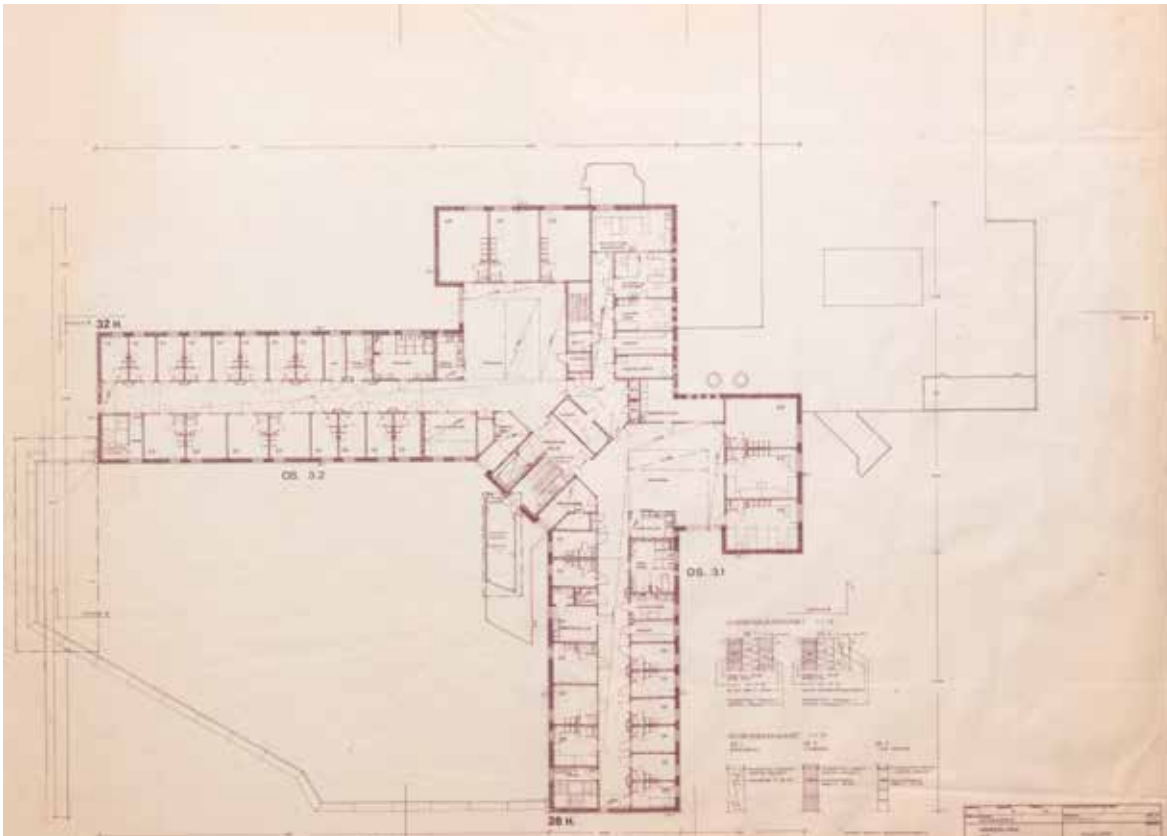
11.9.1985 Veli Paatelan päiväämä ja allekirjoittama vankisairaalan kolmannen kerroksen pääpiirustus. Kansallisarkisto.
