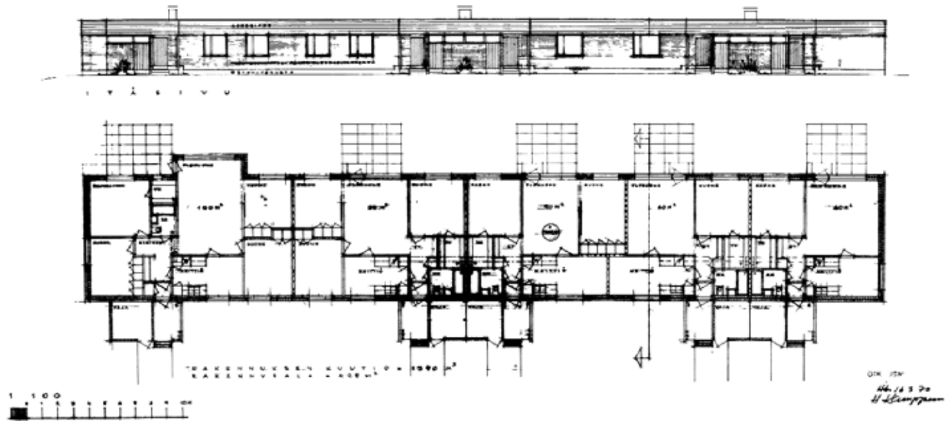
Henno Kamppurin julkisivu- ja pohjapiirustukset, jotka on päivätty 16.3.1970.
