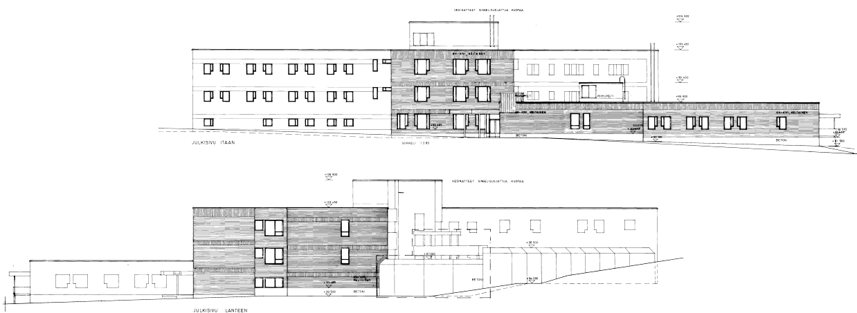
Vankisairaalan itä- ja länsijulkisivut. Veli Paatelan piirustus 11.9.1985
