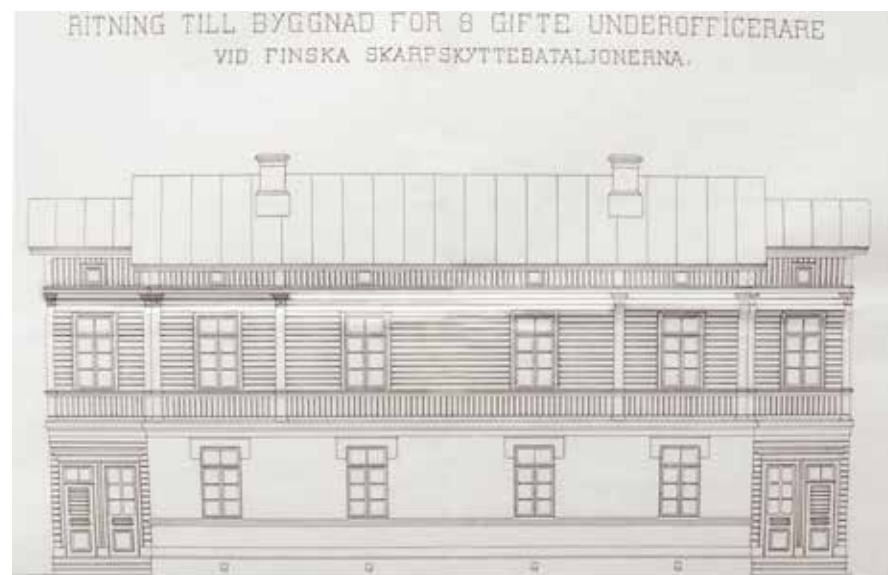
Asuinrakennuksen julkisivupiirros Kansallisarkiston kokoelmista. Samalla tyyppi-piirustuksella tehtiin asuinrakennuksia myös muille kasarmialueille.KA.
