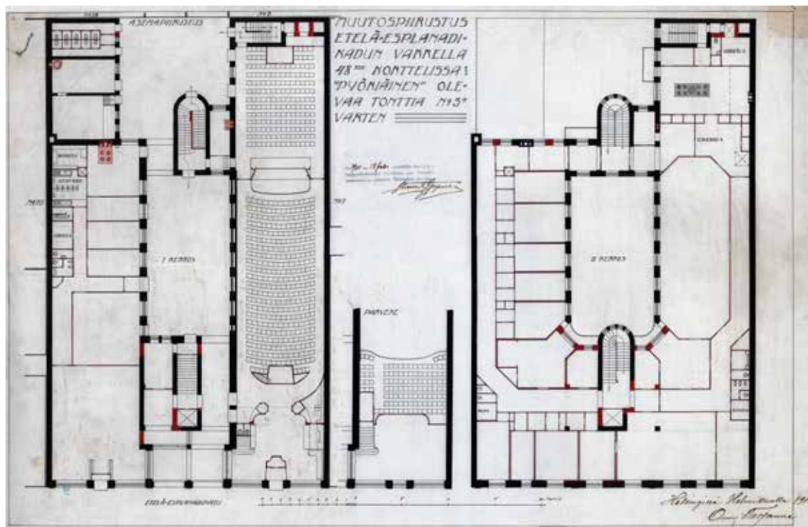
Toteutuspiirros. Ensimmäisen ja toisen kerroksen pohjakuvat. Ensimmäisen kerroksen itäsiivessä oli ravintolasali, pianohuone ja keittiö. Länsisiivessä oli kaksisalininen elokuvateatteri. Molempiin oli oma sisäänkäynti kadulta. Keskellä oli hotellin sisäänkäynti ja pääsy porttikäytän kautta sisäpihoille. Toinen kerros oli varattu ravintolasaliksi, kabineteiksi ja muutamalle hotelli-huoneelle. Eteläpäädyssä oli ravintolan keittiö. Onni Tarjanne, 1910. HKA.
