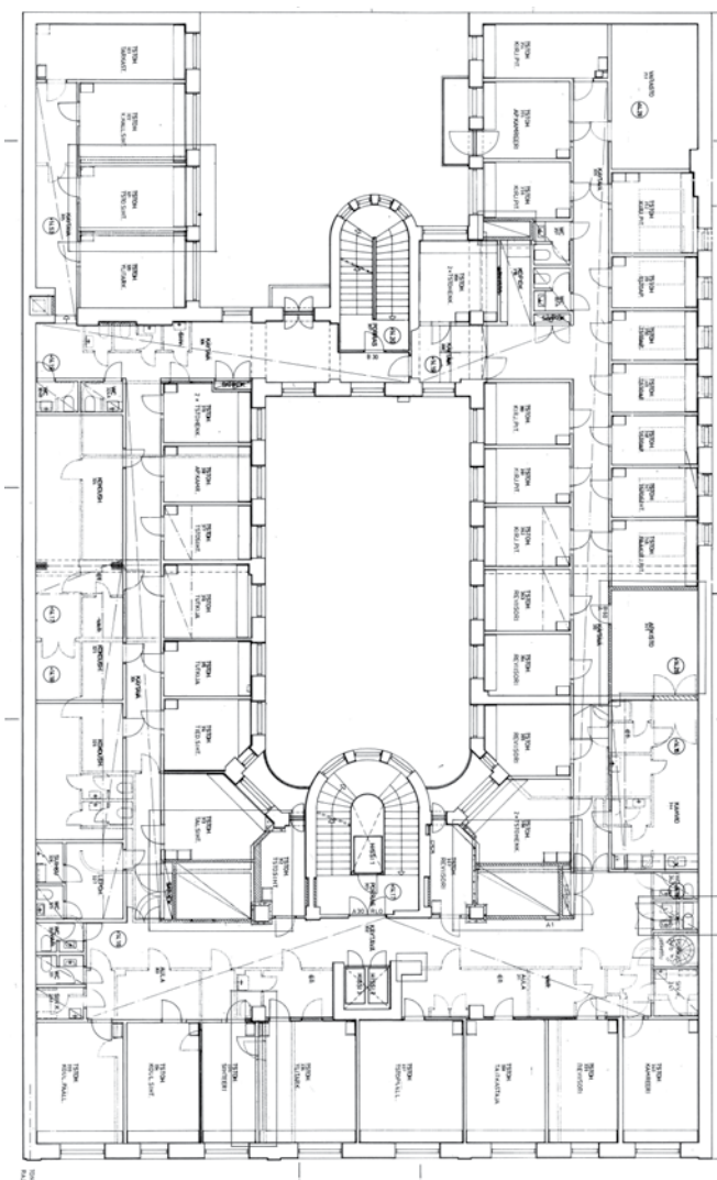
Pääpiirros. Kolmannen kerroksen pohjapiirros. Keskikäytävä-ratkaisu vietiin peruskorjauksessa järjestelmällisesti toimistokerroksissa läpi ja toimistohuoneiden vakiokoko oli yhden hengen huone. Arkkitehtitoimisto Eva ja Jaakko Paatela, 1982. SK.
