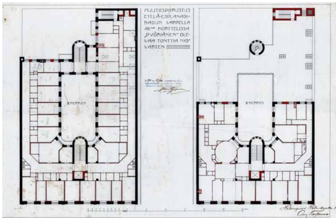
Toteutuspiirros, kolmannen ja neljännen kerroksen pohjakuvat. Kolmas kerros oli hotellikäytössä ja aputiloissa oli kattoikkunat. Neljäs kerros sisälsi hotellihuoneita ja muutaman asuinhuoneiston. Sivusiipien päädyistä oli pääsy suurelle kattoterssille. Onni Tarjanne, 1910. HKA.
