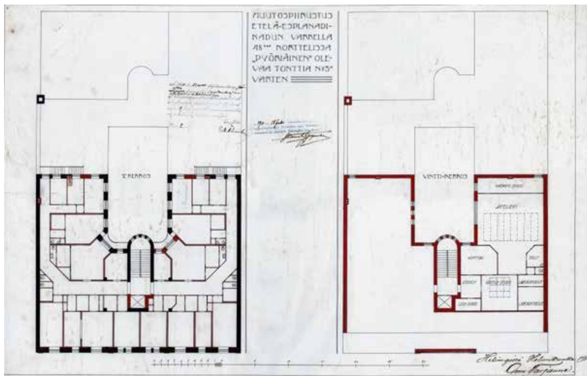
Toteutuspiirros, viidennen kerroksen ja vinttikerroksen pohjakuvat. Viides kerros sisälsi hotellihuoneita ja yhden asunnon. Vintillä oli valokuvausateljee kattoikkunoineen. Ateljeen sisäpihanpuoleinen ikkuna hyödynnettiin vuoden 1934 korotuksessa. Onni Tarjanne, 1910. HKA.
