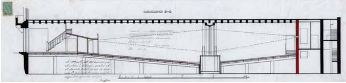
Pääpiirustus, teatterin leikkauspiirros. Piirustus täydentää saman vuoden pääpiirustussarjaa. Onni Tarjanne, 1909. HKA.
