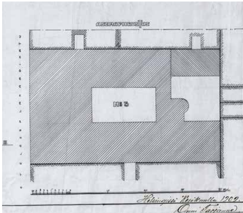
Onni Tarjanteen piirtämä asemapiirros vuodelta 1909. U-kirjaimen muotoisen pohjaratkaisun siipiä yhdisti kapea käytävä. Taaemman pihan itäpuolella oli matala piharakennus. Piirustus täydentää saman vuoden pääpiirustussarjaa. HKA.
