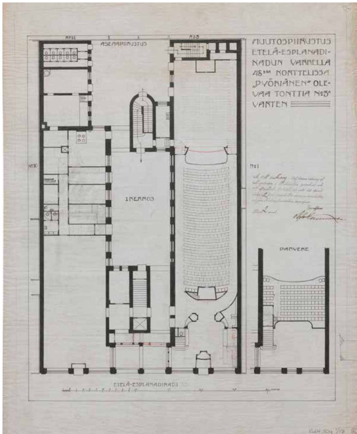
Ensimmäisen kerroksen pohjapiirros; elokuvateatteri muutettuna operettiteatteriksi, 1911. KA.
