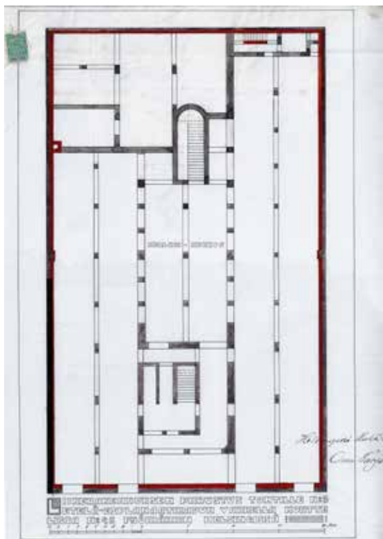
Pääpiirustus, kellarikerroksen pohjapiirros. Kellarikerros ulottui alusta alkaen koko tontin alueelle. Kellarissa oli lähinnä varastotilaa ja teatterisalin alapuoleinen tila oli osin hyvin matala. Onni Tarjanne, 1909. HKA.
