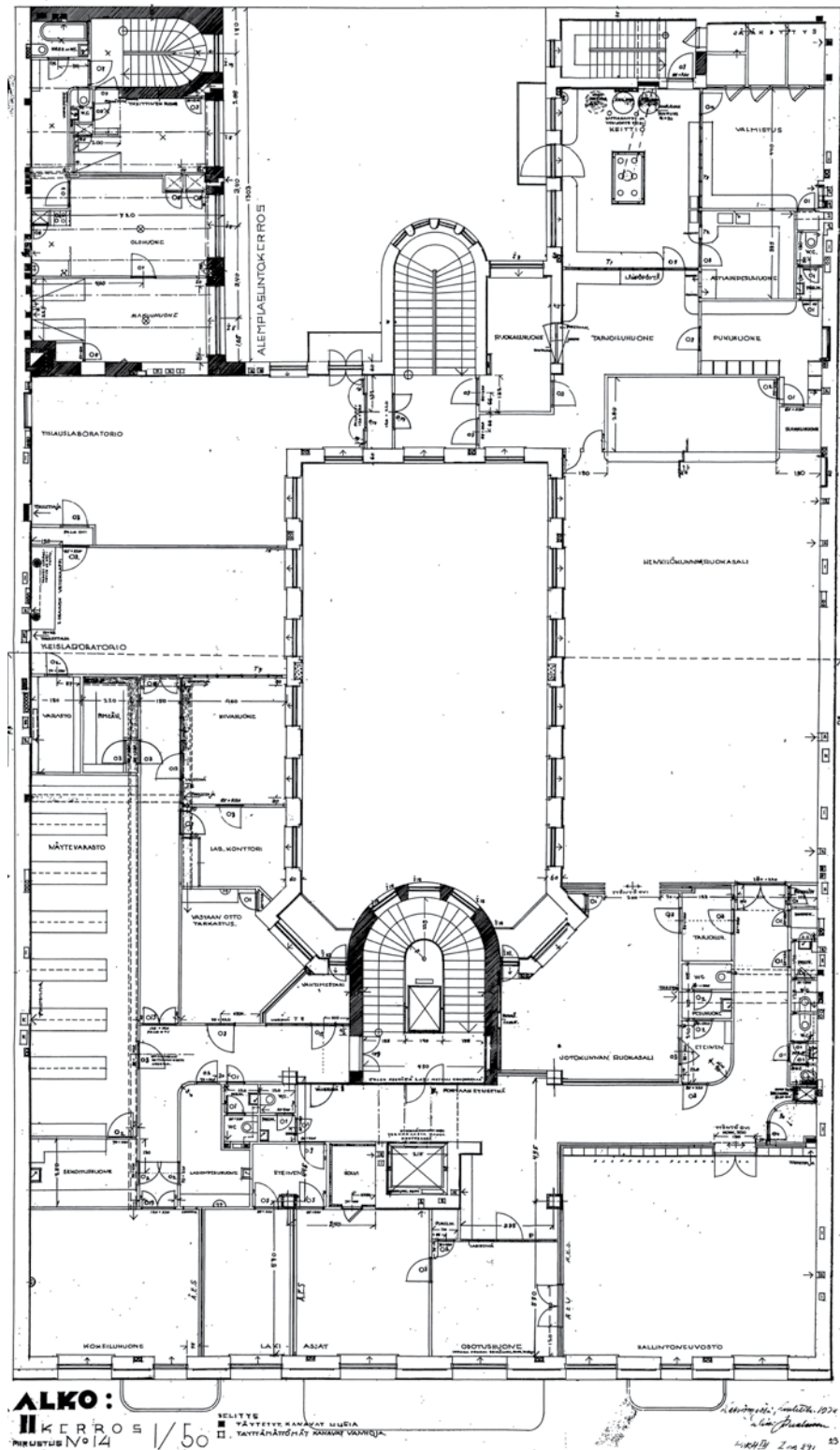
Toiseen kerrokseen sijoitettiin edustustilat, tuotekehityslaboratorio maisteluhuoneineen ja hallintoneuvoston kokoushuone. Pohjapiirros, P. E. Blomstedt / Elias Paalanen, 1934. KA.
