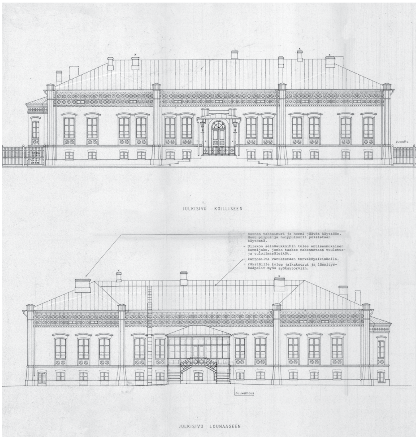
1980-luvun lopulla laadittu peruskorjaussuunnitelma julkisivuista. Yllä koillisjulkisivu, alla lounaisjulkisivu. Piirustusta on rajattu. Senaatti-kiinteistöt.
