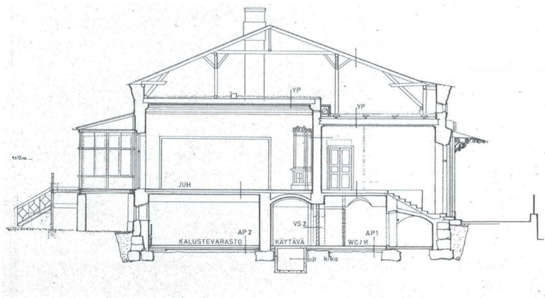
1980-luvun lopulla laaditun peruskorjaussuunnitelman leikkauspiirustus, jossa on esitetty korjaustoimet. Senaatti-kiinteistöt.
