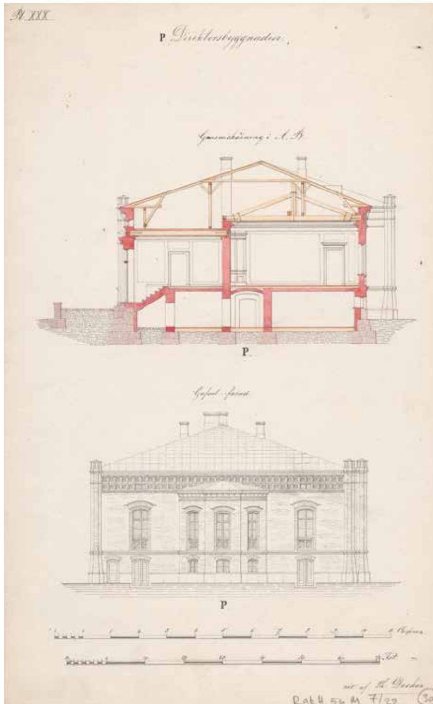
Theodor Deckerin päiväämätön piirustus kadettikoulun johtajan asuinrakennuksen kaakkoisjulkisivusta ja rakennuksen leikkaus. Kansallisarkisto.
