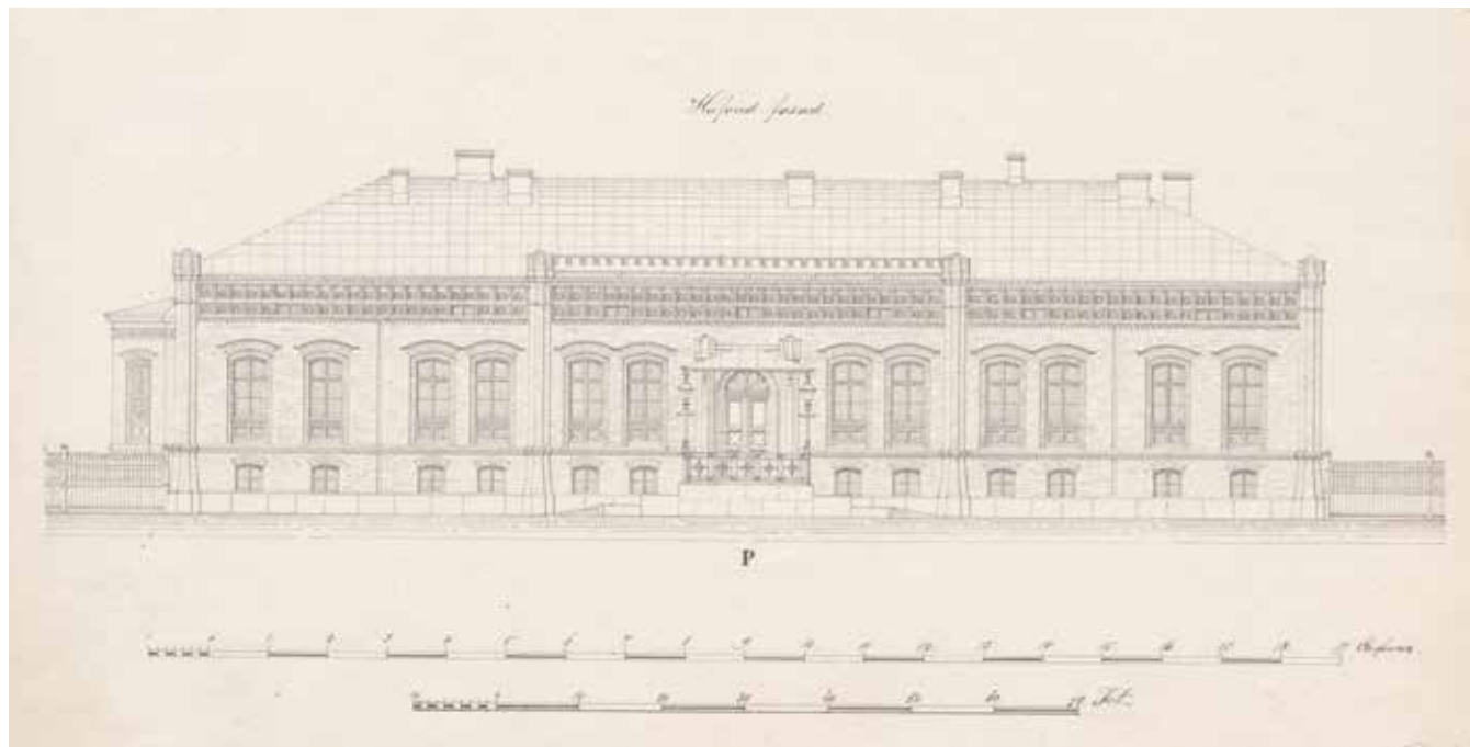
Theodor Deckerin päiväämätön piirustus kadettikoulun johtajan asuinrakennuksen pääjulkisivusta. Rakennus toteutettiin kyseisen suunnitelman mukaan. Kansallisarkisto.
