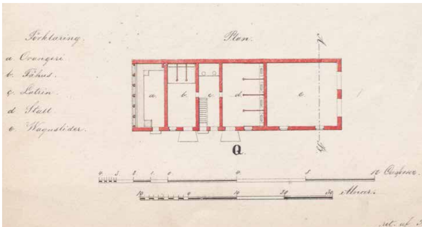
Theodor Deckerin päiväämätön piirustus kadettikoulun johtajan asuinrakennuksen yhteyteen rakennetusta talousrakennuksesta. Pohjapiirustus. Piirustusta on rajattu. Kansallisarkisto.
