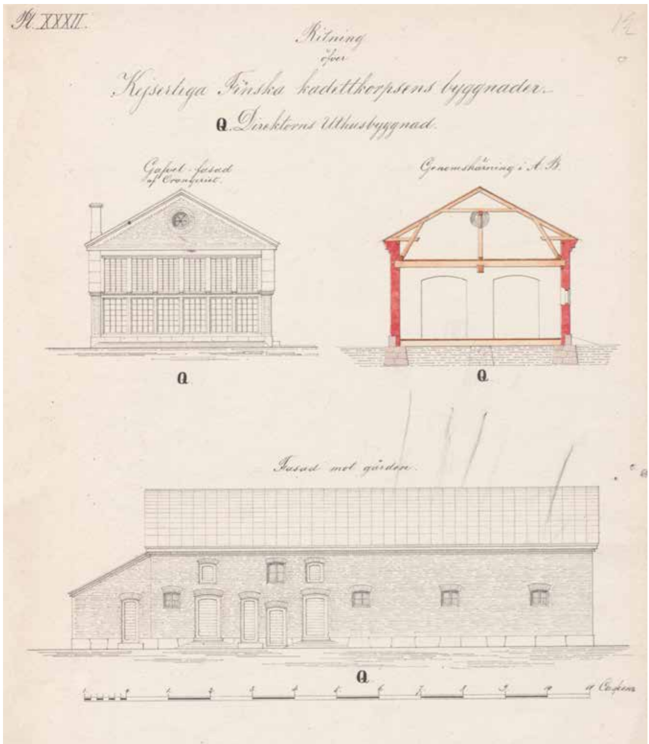
Theodor Deckerin päiväämätön piirustus kadettikoulun johtajan asuinrakennuksen yhteyteen rakennetusta talousrakennuksesta. Yllä lounaisjulkisivu ja leikkaus, alla kaakkoisjulkisivu. Piirustusta on rajattu. Kansallisarkisto.
