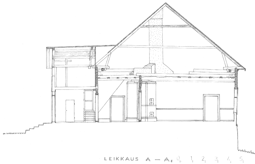
Leikkaus pääkuistin ja ruokasalin poikki. Piirtänyt 1967 Reino Peltonen. MVA.
