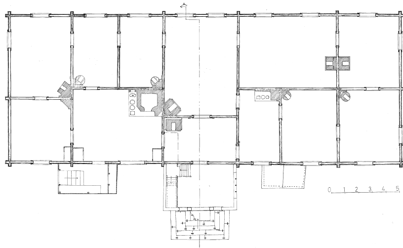
Mittauspiirros 1977, MVRHO.
