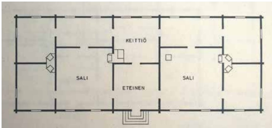
Pohjapiirros 1738, MVRHO.
