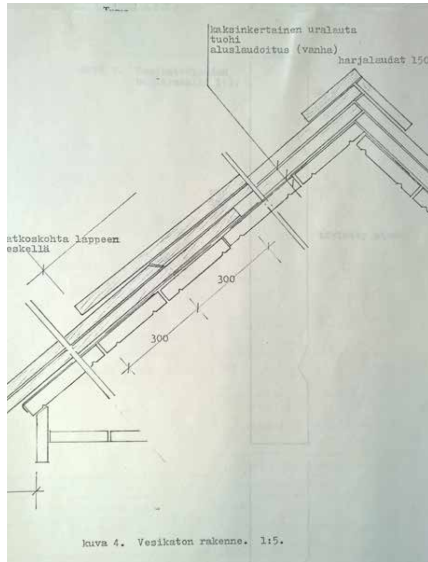
Panu Kailan periaatesuunnitelma lautakatosta. Kunnan mukaan järjestetyt asiakirjat. MVRHO.
