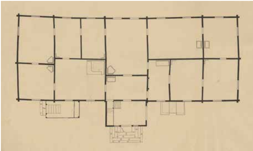
Pohjapiirros 1927, T. Strömberg ja E. Waskinen. TKK/Aalto.
