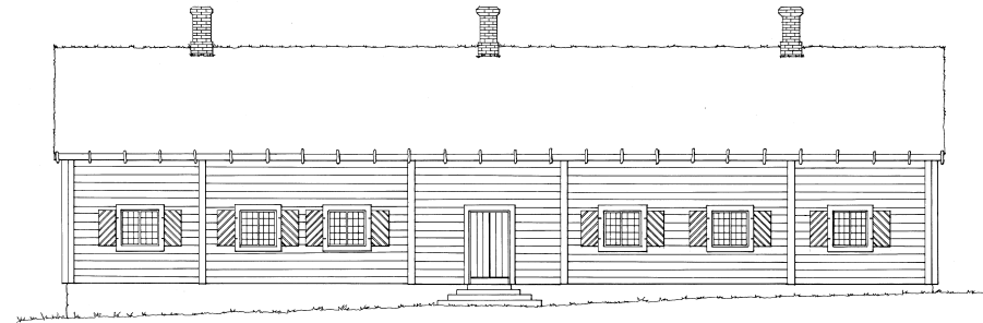
Pääjulkisivu 1738, MVRHO.
