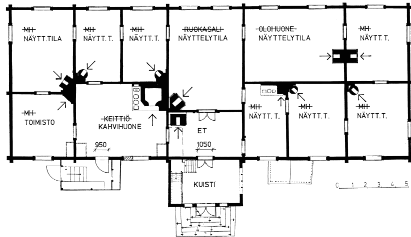
Tilasuunnitelma 1978, MVRHO.
