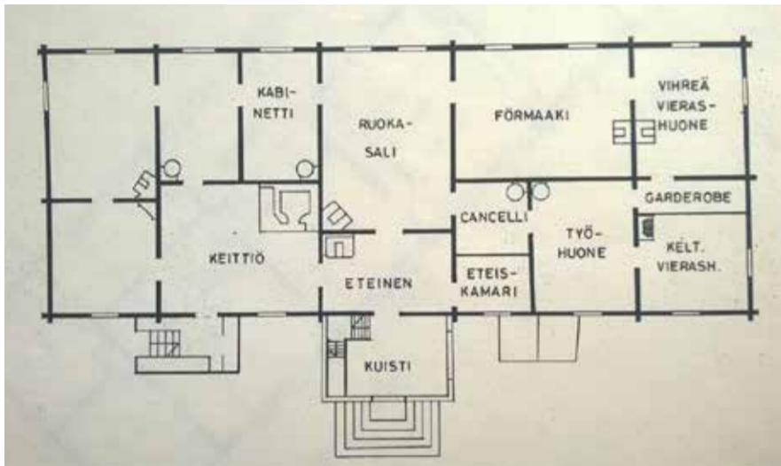
Pohjapiirros 1840, MVRHO.
