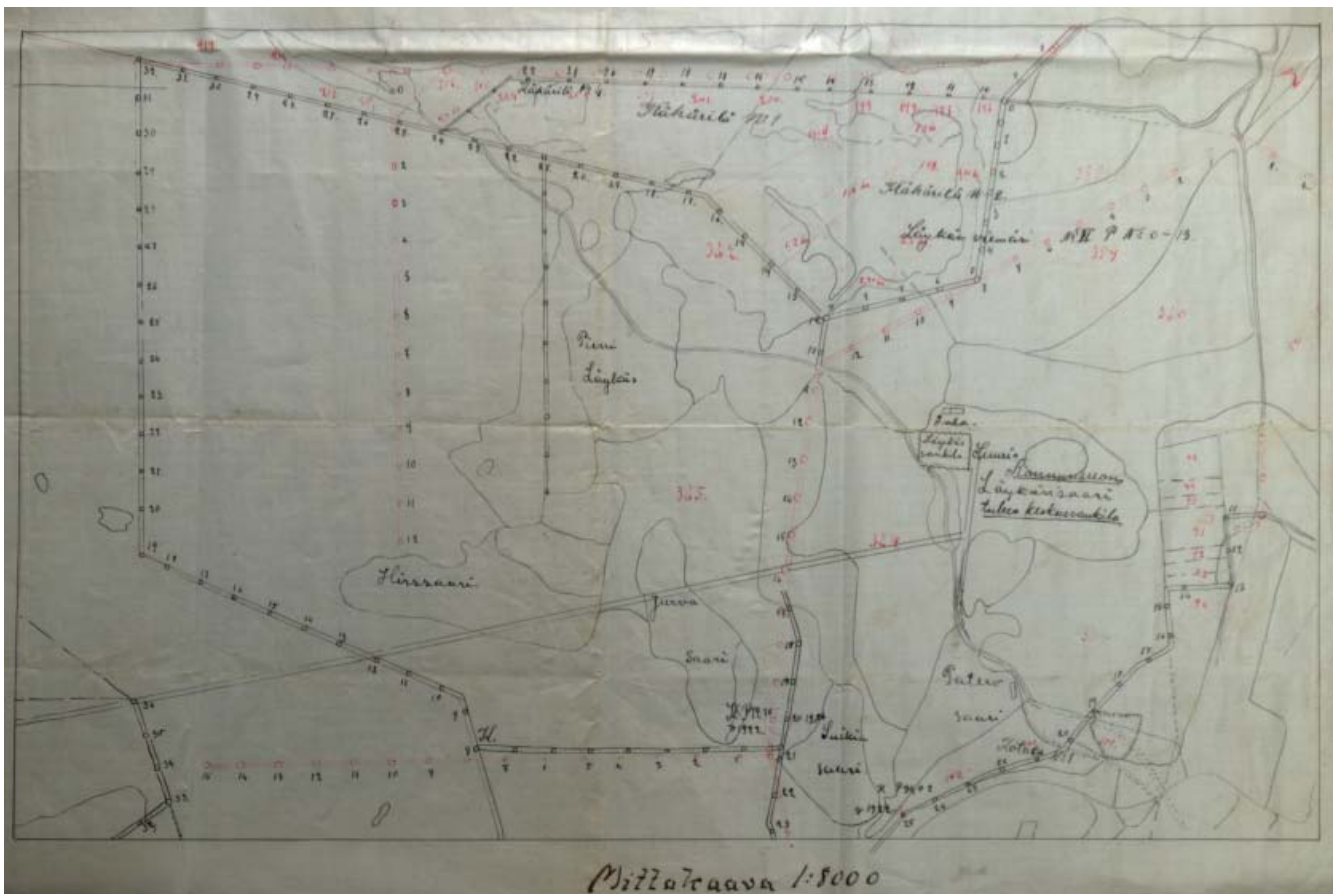
Konnausuo kuivatuksen suunnitelma. Kuivatussuunnitelman laati Vilho Mäkinen 1913. Kuvan kartta on nähtävästi piirretty 1920-luvun alussa, sillä karttaan on merkitty kenttäradan linja Tuomojalta Lyykkään ja Lyykänsaareen teksti "Konnausuo tuleva keskusvankila"
