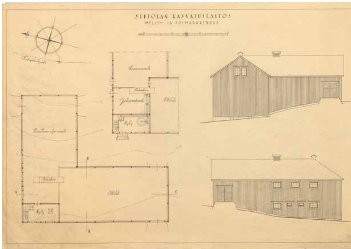
Mylly- ja puimarakennuksen julkisivut etelään ja pohjoiseen sekä pohjapiirrokset. Piirustus on todennäköisesti 1920-luvulta. KA.
