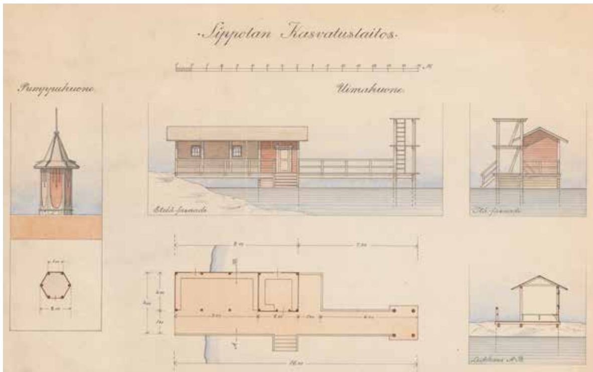
Kartanon pihapiirin pumppuhuoneen (Ä) julkisivu ja pohjapiirros, uimahuoneen (U) julkisivut etelään ja itään, pohjapiirros sekä leikkaus A-B. Yleisten rakennusten ylihallituksen arkkitehdit Th. Granstedt ja Hugo Lindberg, 9.9.1910. Kosjärven uimahuone oli yksikerroksinen, harjakattoinen, punamullattu puurakennus, johon liittyi laituri ja sen päässä kaksikerroksinen puinen hyppytorni. Pumppu- ja uimahuonetta ei ole enää olemassa.KA.
