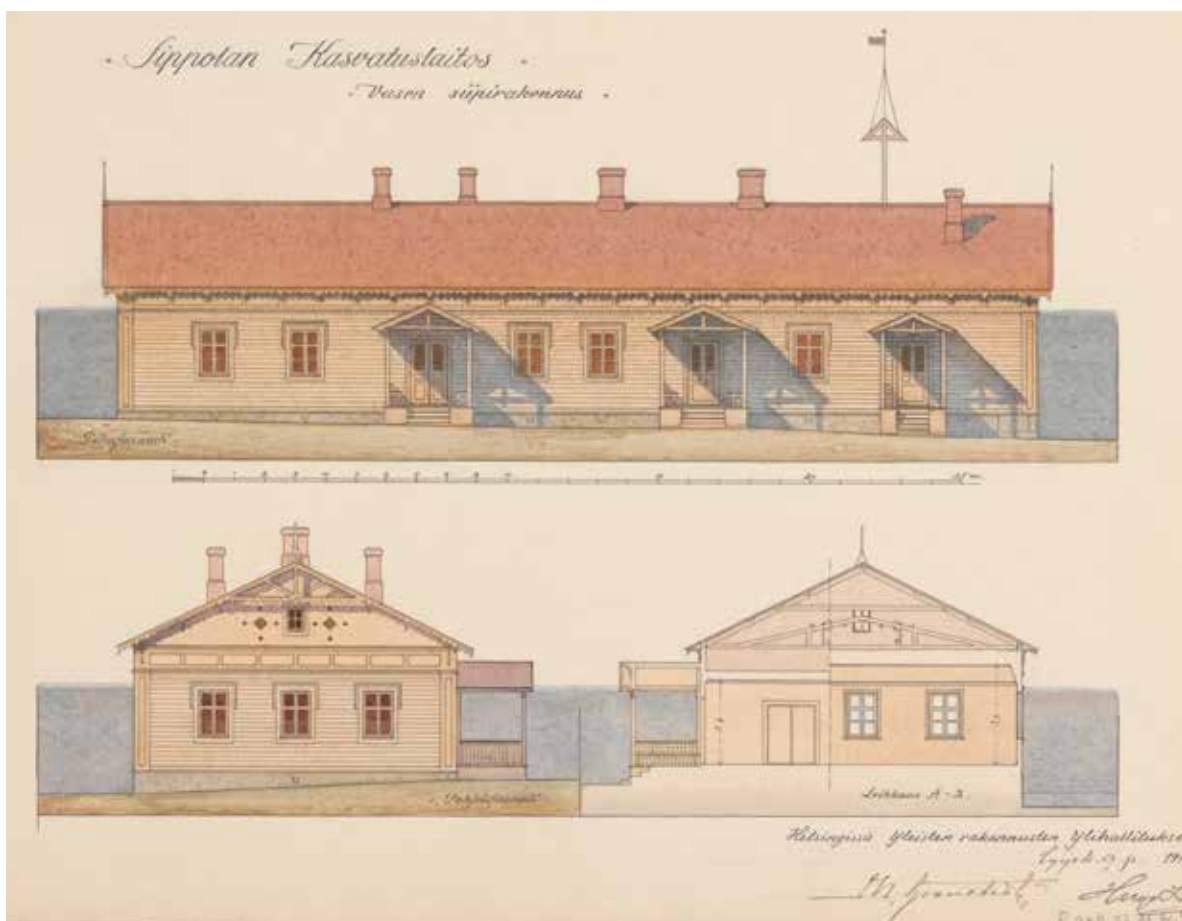
Vasemman siipirakennuksen julkisivut länteen ja pohjoiseen sekä leikkaus A-B. Yleisten rakennusten ylihallituksen arkkitehdit Theodor Granstedt ja Hugo Lindberg, 9.9.1910. Rakennus oli peräisin 1800-luvulta, mutta sitä laajennettiin kasvatustaitoksen ottaessa rakennuksen käyttöönsä. KA.
