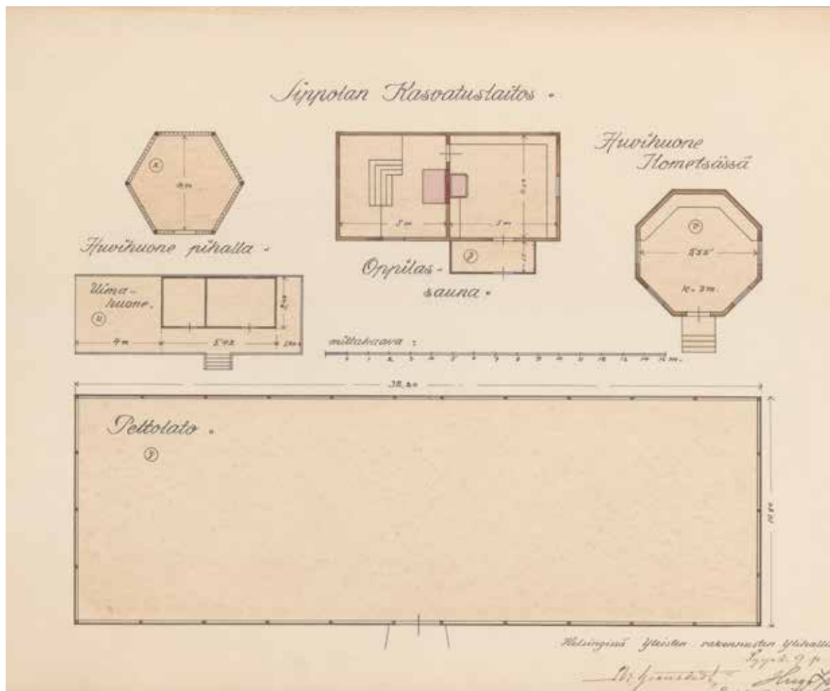
Pihan huvihuoneen (X), oppilassaunan (J), Ilometsän huvihuoneen (V), Kosjärven rannan uimahuoneen (U) ja peltoladon (Y) pohjapiirrokset. Yleisten rakennusten ylihallituksen arkkitehdit Th. Granstedt ja Hugo Lindberg, 9.9.1910. Ilometsän huvihuone siirrettiin myöhemmin vuonna 1926 Korpivaaraan retkimajaksi. KA.
