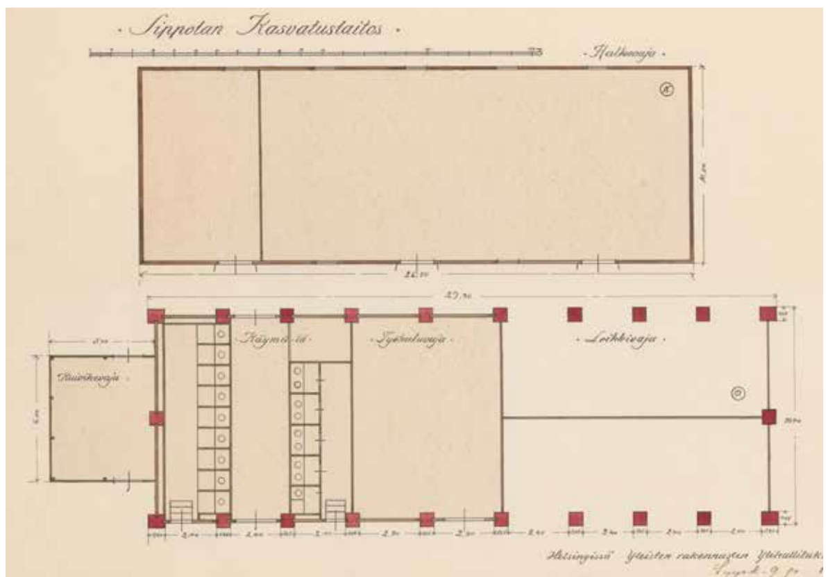
Halkovajan (N, entinen kartanoaikainen talli) sekä käymälä/vajarakennuksen (O) pohjapiirrokset. Yleisten rakennusten yllähdituksen arkkitehdit Th. Granstedt ja Hugo Lindberg, 9.9.1910. Vaja- ja käymälärakennuksen sisätiloja muutettiin 1910. Kumpikin rakennus on purettu 1900-luvulla. KA.
