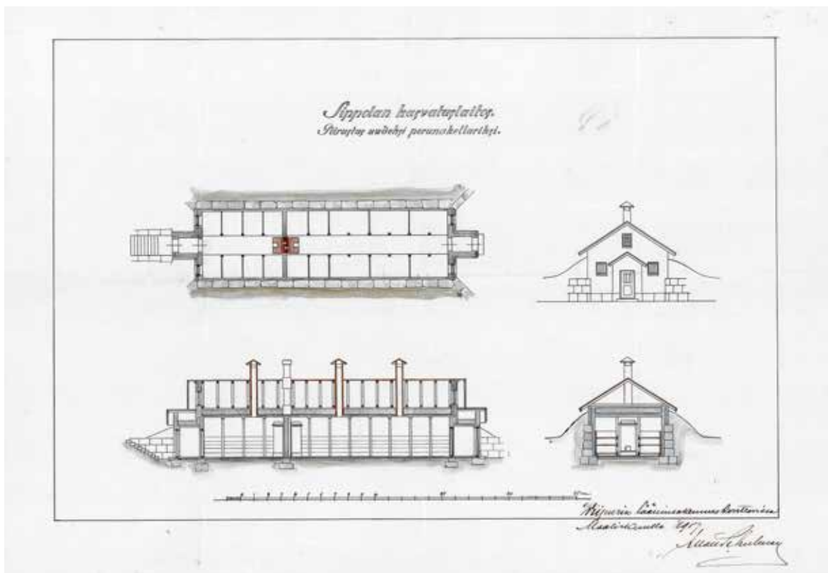
Sippolan kasvatuslaitoksen perunakellarin pohjapiirros, leikkaukset ja päätyjulkisivu. Viipurin lääninrakennuskonttorissa maaliskuussa 1917, suunnittelijana Allan Schulman. Kivirakenteisessa kellarissa sijaitsi kaksi uunia ja puisia väliseiniä. Rakennus on sittemmin purettu. Alkuperäispiirustus on päärakennuksen seinällä. SiA.
