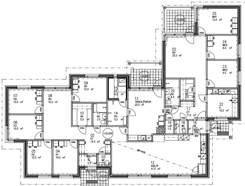
Perhekoti, Talo I. Ensimmäinen kerros. Arkkitehtitoimisto Karjalainen Juola Salo. 8.12.1989. Sk Kouvola.
