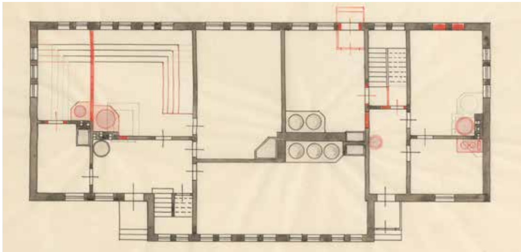
Saunarakennuksen ensimmäisen kerroksen pohja. Yleisten rakennusten ylihallitus. Piirustus on päiväämätön muutospiirustus. Muutospaikat on merkitty punaisella. KA.
