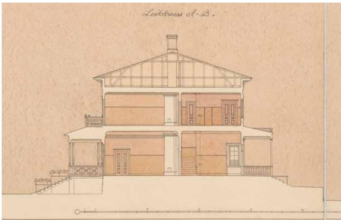
Päärakennuksen leikkaus A-B. Yleisten rakennusten ylihallituksen arkkitehdit Theodor Granstedt ja Hugo Lindberg, 9.9.1910. KA.
