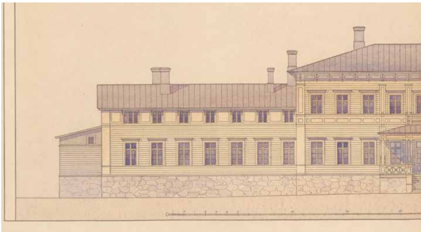
Päärakennuksen julkisivu etelään eli puiston puolelle. Yleisten rakennusten ylihallituksen arkkitehdit Theodor Granstedt ja Hugo Lindberg, 9.9.1910. KA.
