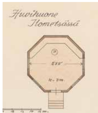
Ilometsän huvihuoneen pohjapiirros. Yleisten rakennusten ylihallituksen arkkitehdit Th. Granstedt ja Hugo Lindberg, 9.9.1910. KA.
