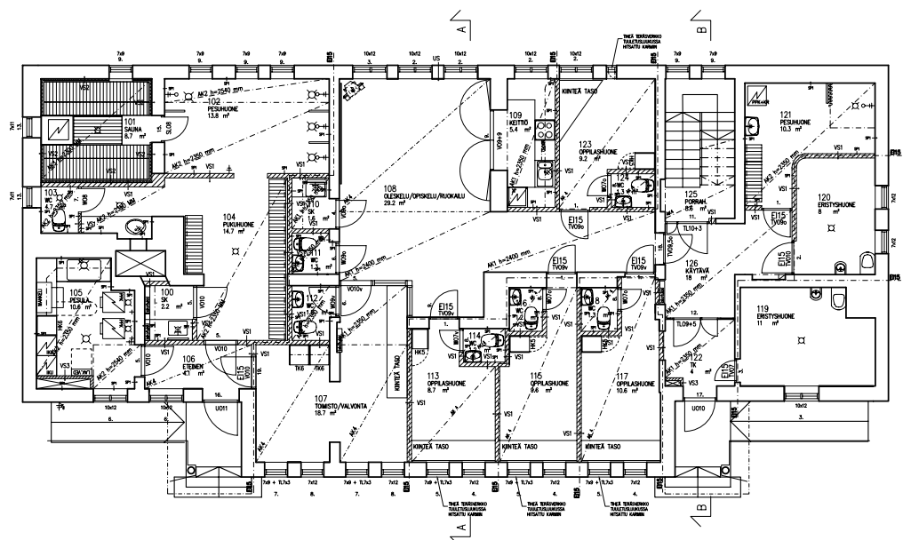
Erityishuollon osaston (entisen sauna- ja pesularakennuksen) ensimmäisen kerroksen muutospiirustus. Arkkitehtitoimisto Heikki Kirjalainen, 12.9.2003. Sk Kouvola.
