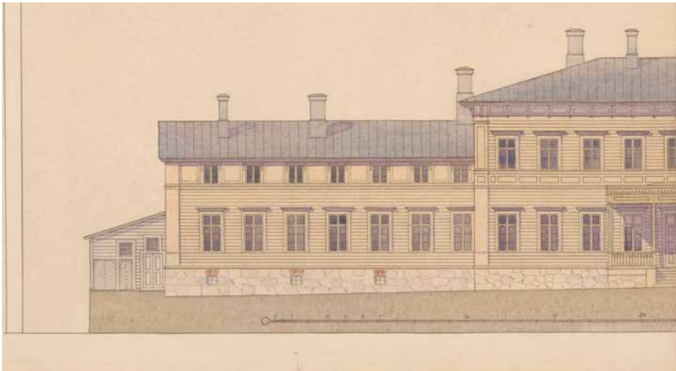
Päärakennuksen julkisivu pohjoiseen. Yleisten rakennusten ylihallituksen arkkitehdit Theodor Granstedt ja Hugo Lindberg, 9.9.1910. KA.
