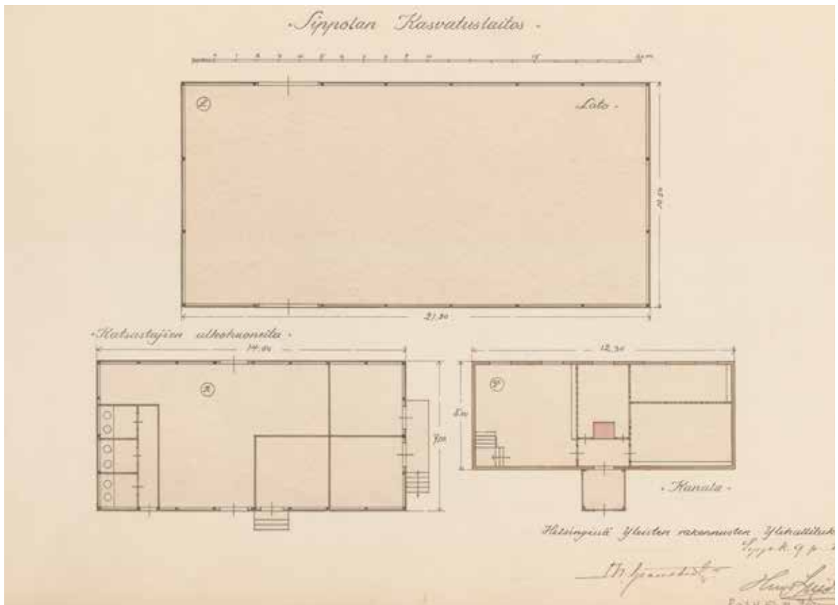
Kartanovaiheen rakennuksia: ladon (L), katsastajien ulkokuoneiden (R) sekä kanalan (P) pohjapiirrokset. Yleisten rakennusten yllähdituksen arkkitehdit Th. Granstedt ja Hugo Lindberg, 9.9.1910. Rakennuksia ei enää ole olemassa. KA.
