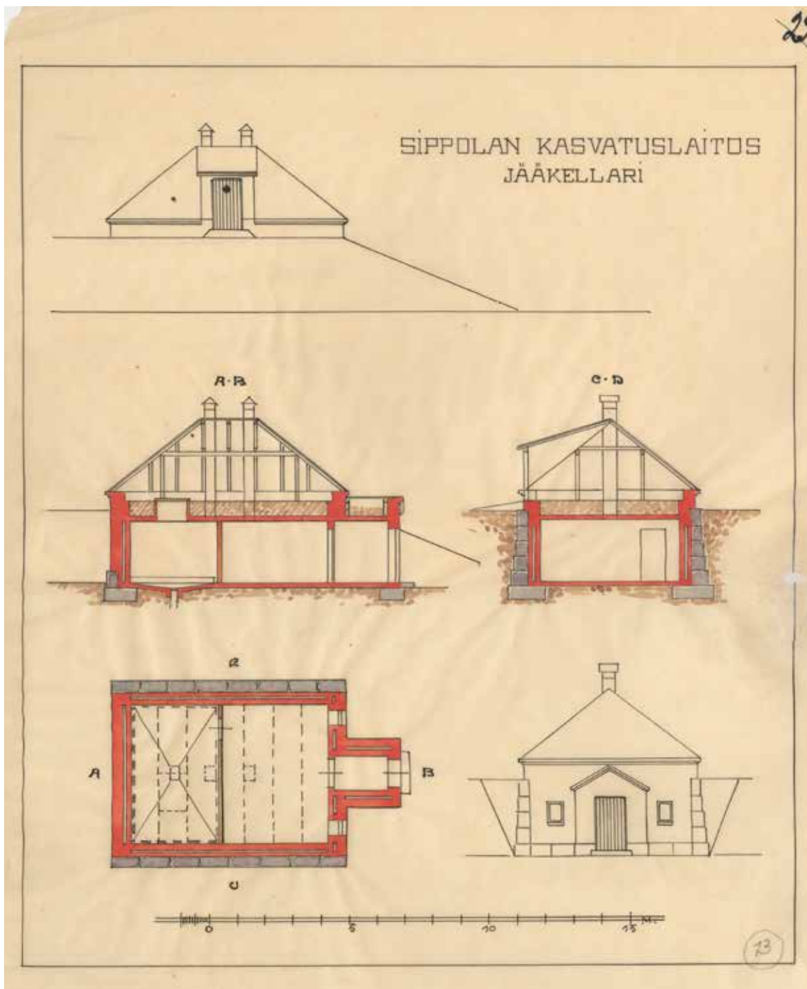
Jääkellarin julkisivut, leikkaukset A-B ja C-D sekä pohjapiirros. Piirrosta ei ole päivätty eikä allekirjoitettu, mutta se on todennäköisesti 1909-1910. Kellari on purettu myöhemmin 1900-luvulla. KA.
