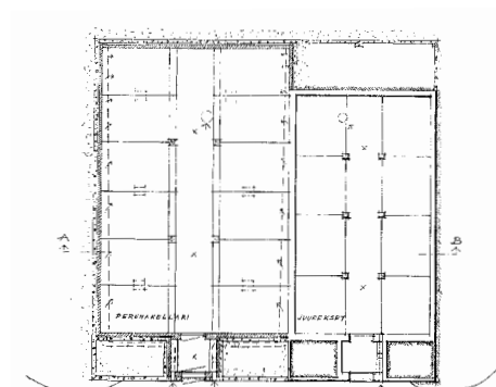
Kellarin pohja. Suunnittelija: Vuorinen. 1961. Sk Kouvola.
