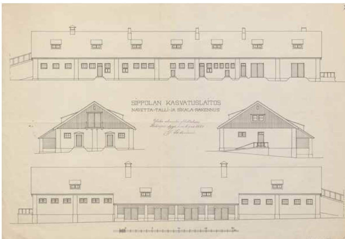
Uudisrakennusvaiheen julkisivut. Y. Sadeniemi, Yleisten rakennusten ylihallitus. 6.9.1924. KA.
