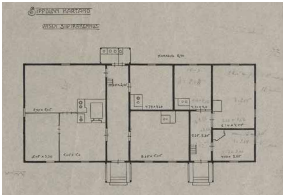
Vasemman siipirakennuksen pohjapiirros. Yleisten rakennusten ylihallituksen arkkitehdit Theodor Granstedt ja Hugo Lindberg, todennäköisesti vuodelta 1909. Piirustus esittää rakennuksen kartanovaiheen tilannetta ennen laajennus- ja muutostöitä. KA.
