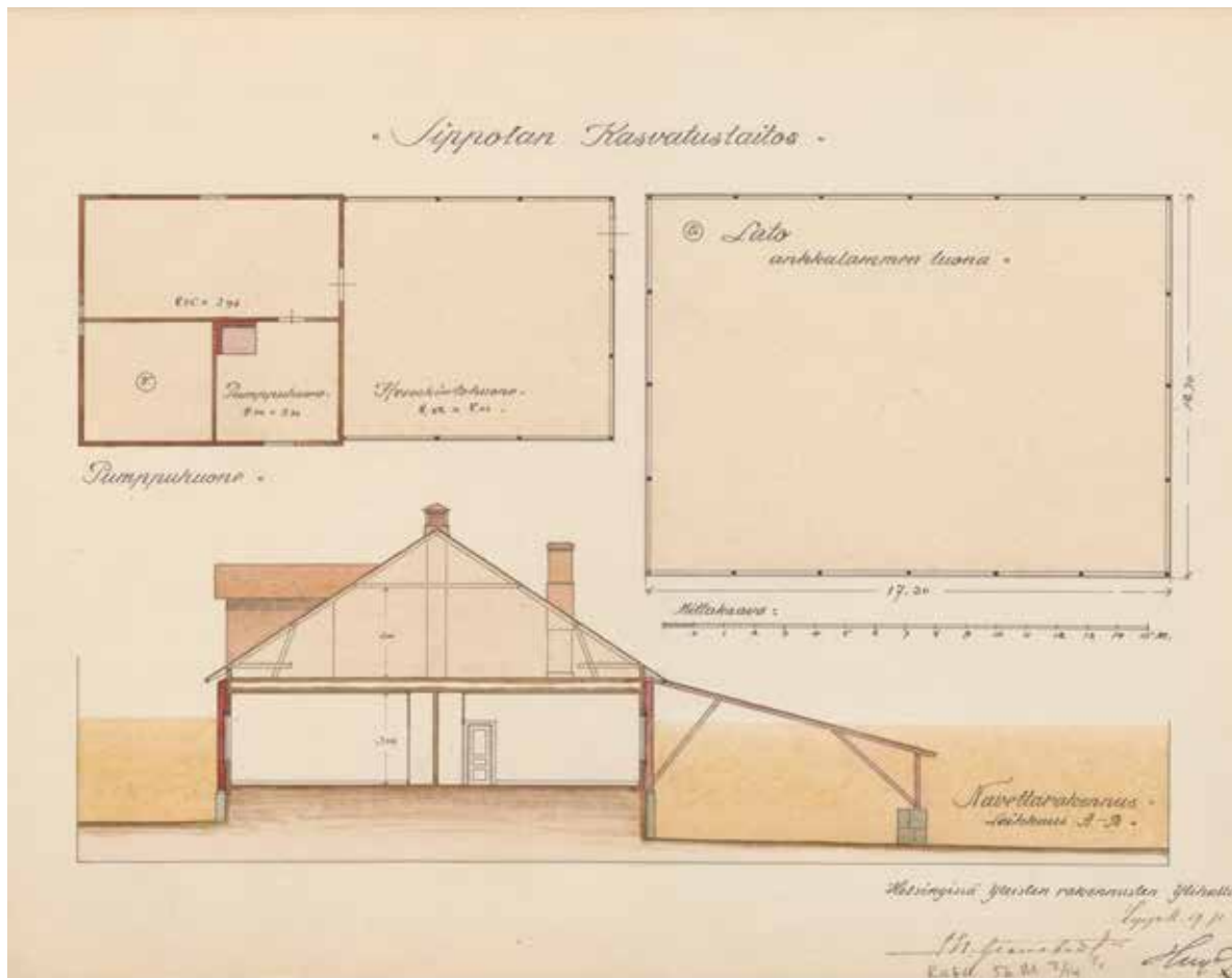
Pumppuhuoneen ja ankkalammen viereisen ladon pohjapiirroksiset sekä navettarakennuksen leikkaus A-B. Yleisten rakennusten ylihallituksen arkkitehdit Th. Granstedt ja Hugo Lindberg, 9.9.1910. Kaikki rakennukset on sittemmin purettu myöhemmin 1900-luvulla. Navettarakennus purettiin uuden navetan alta 1920-luvulla. KA.
