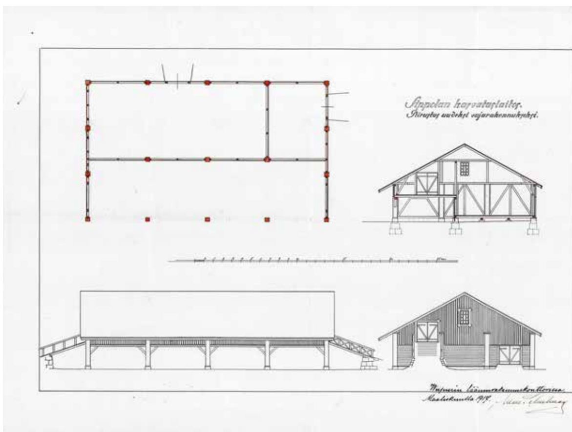
Kasvatuslaitoksen uuden vajakennuksen pohjapiirros, leikkaus ja julkisivut. Viipurin lääninrakennuskonttorissa maaliskuussa 1917 allekirjoittanut Schulman. Alkuperäispiirustus on päärakennuksen seinällä. SiA.
