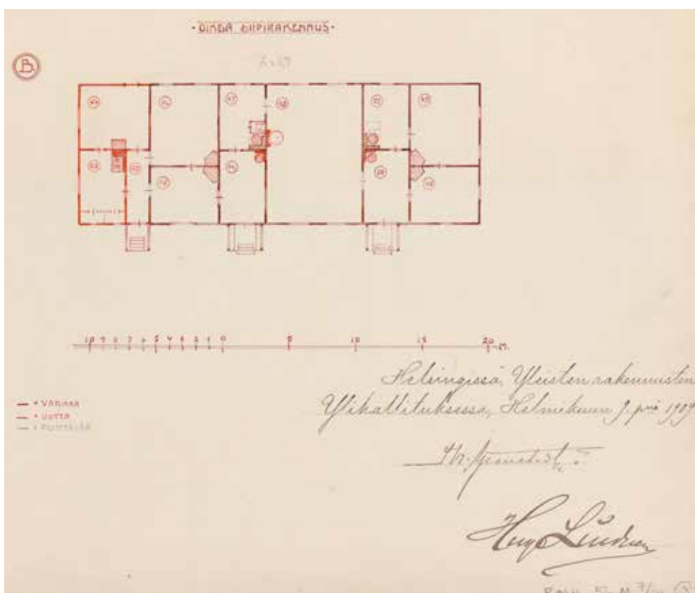
Oikean siipirakennuksen pohjapiirros. Yleisten rakennusten ylihallituksen arkkitehdit Theodor Granstedt ja Hugo Lindberg, 9.2.1909. Rakennus oli peräisin 1800-luvulta, mutta sitä laajennettiin kasvatustilakoulun ottaessa rakennuksen käyttöönsä. Laajennusosa on kuvan vasemmanpuoleinen kirkkaanpunaisella piirretty päätyosuus. KA.
