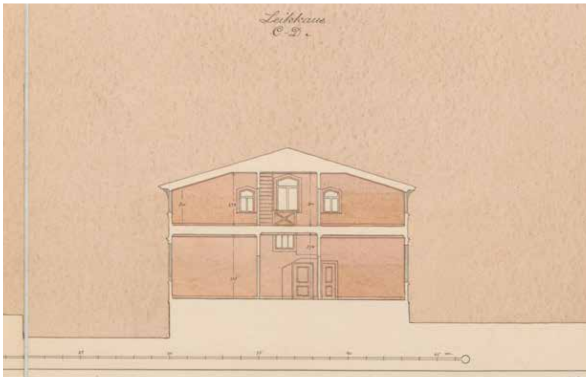
Päärakennuksen leikkaus C-D. Yleisten rakennusten ylihallituksen arkkitehdit Theodor Granstedt ja Hugo Lindberg, 9.9.1910. KA.
