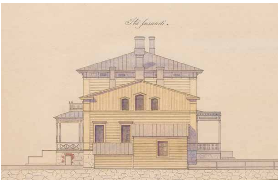
Päärakennuksen päätyjulkisivu itään. Yleisten rakennusten ylihallituksen arkkitehdit Theodor Granstedt ja Hugo Lindberg, 9.9.1910. KA.
