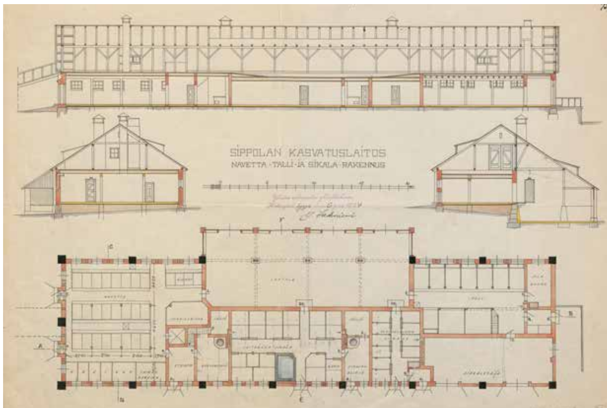
Sippolan kasvatustaitoksen navetta-, talli- ja sikalarakennuksen uudisrakennusvaiheen leikkaukset ja pohjapiirros. Y. Sadeniemi, Yleisten rakennusten ylihallitus. 6.9.1924. KA.
