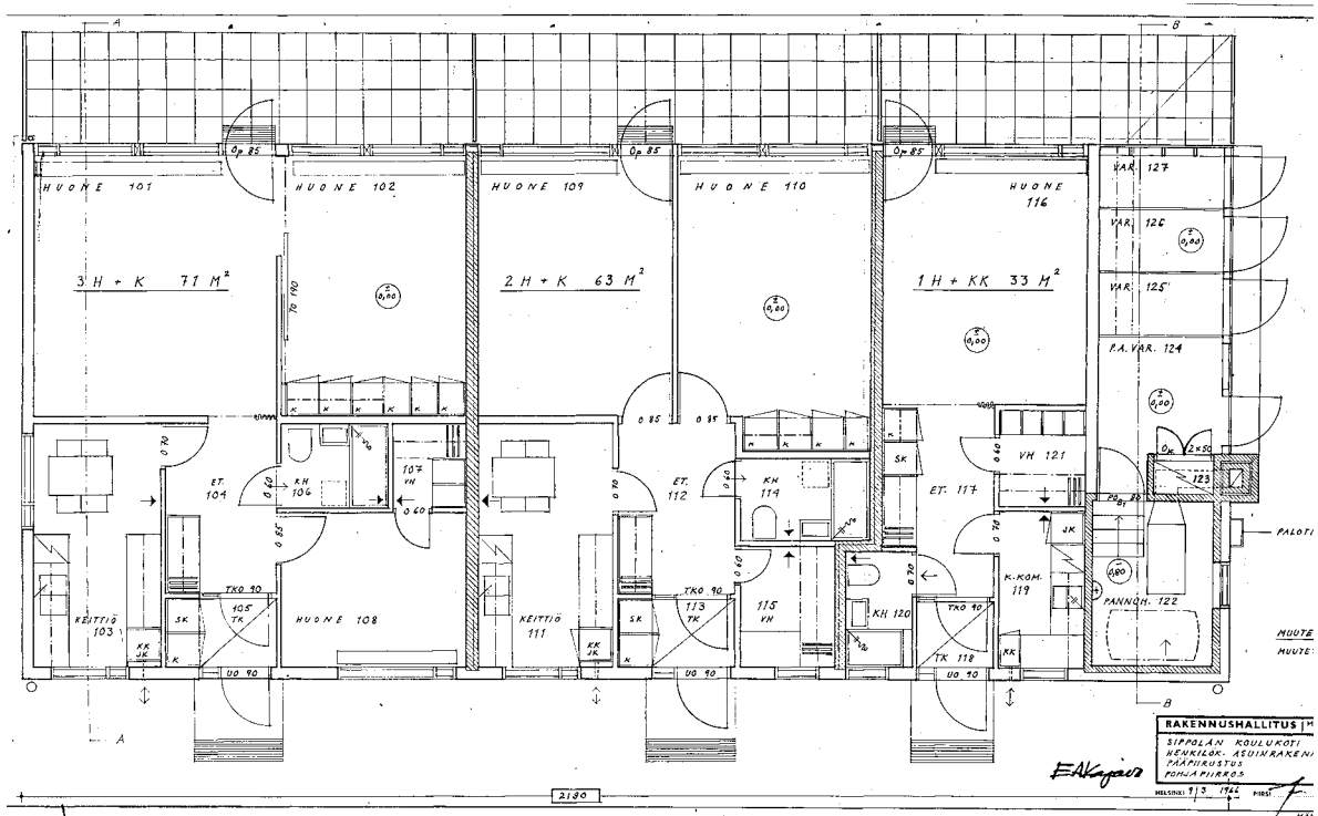
Henkilökunnan asuinrakennus Mäntylän pohjapiirros. 9.3.1966. Arkkitehti J. Kosonen ja E.A. Kajava. Rakennushallitus. Sk Kouvola.
