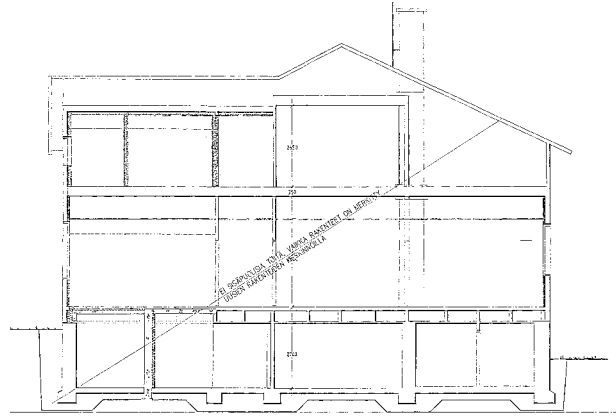
Päärakennuksen muutostöiden leikkaus A-A. Arkkitehtitoimisto Heikki Kirjalainen, 25.5.2001. Sk Kouvola.
