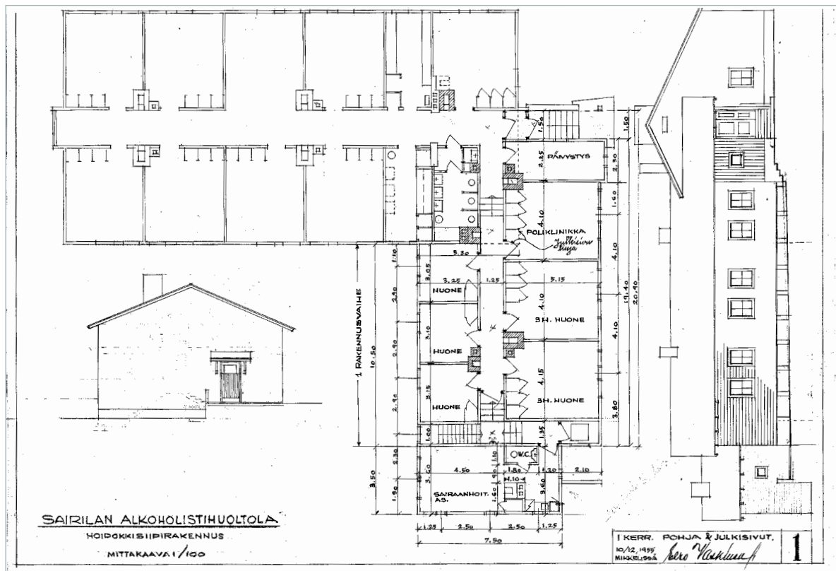
Sairilan alkoholistihuoltolaa varten rakennettiin vuonna 1955 siipirakennus laajentamalla navetan koillispuolella sijainnutta vanhaa rakennusta. Kuvassa ovat siipirakennuksen pohjapiirustus ja julkisivut. Eero Vaskinen Mikkelissä 10.12.1955. Rakennus purettiin 1980-luvulla, mutta sen kiviperustuksia on edelleen havaittavissa. Siivessä sijaitsi kolme potilashuonetta, päiväystyshuone, poliklinikka, kaksi sairaanhoitajan huonetta, sairaanhoitajan asunto sekä wc-tilat. Sk Mikkeli.
