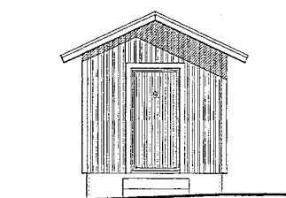
JULKISIVU LÄNTEEN
