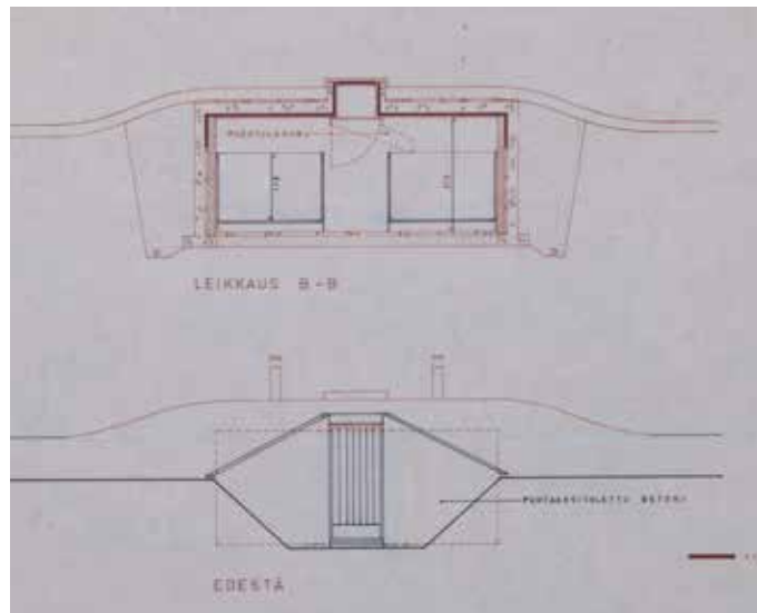
Koulukodin peruna- ja juurikaskellarin uudisrakennusvaiheen leikkaus A-A pohjapiirustus, leikkaus B-B ja julkisivu itään. Arkkitehti Jorma Kosonen, Rakennushallitus, 23.8.1968. Piirustusta on muutettu 14.4.1969. KA.
