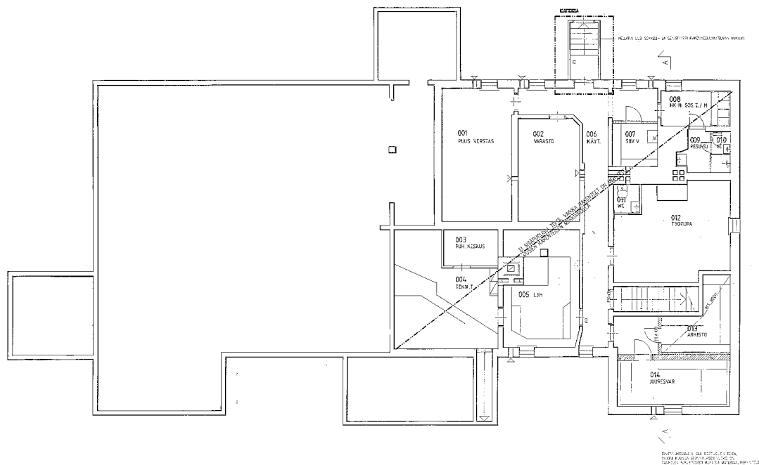
Sairilan koulukodin päärakennuksen muutostöiden kellarikerroksen pohjapiirustus. Arkkitehtitoimisto Heikki Kirjalainen, 25.5.2001. Sk Kouvola.
