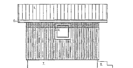
JULKISIVU POHJOISEN
