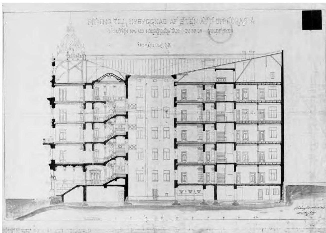
Leikkaus A-B. Axel Höberg 1888. KA.
