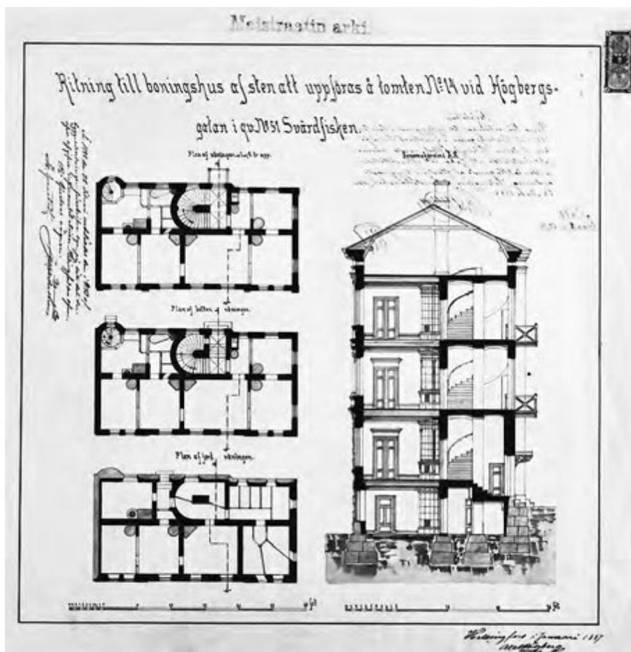
Korkeavuorenkatu 22. Pohjat ja leikkaus. Axel Högborg 1887. HKA SIN.
