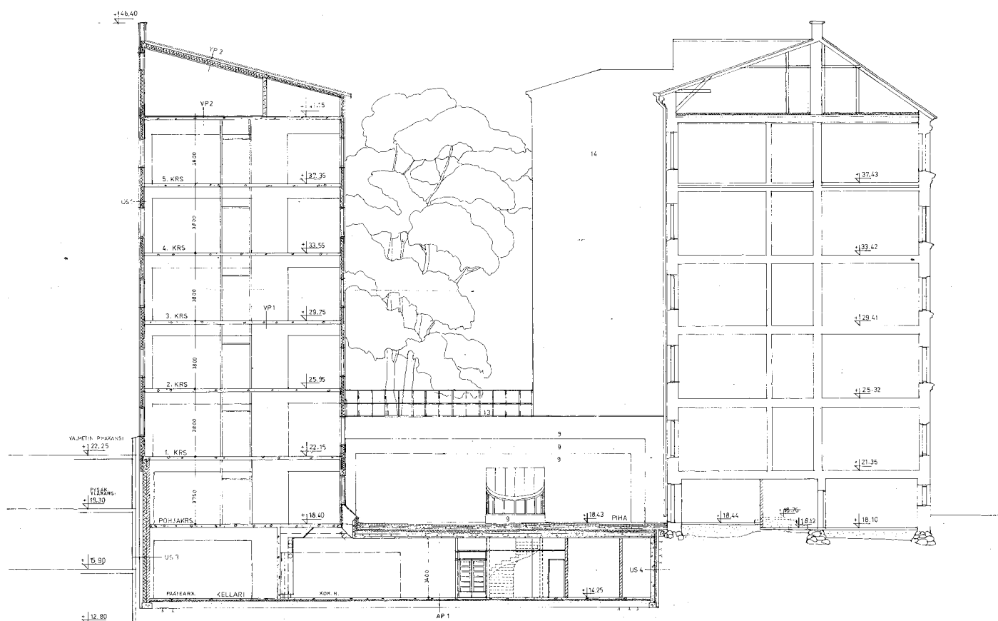
Leikkaus B-B. Arkkitehtuuritoimisto Pirkko ja Arvi Ilonen. 28.9.1989. Sk.
