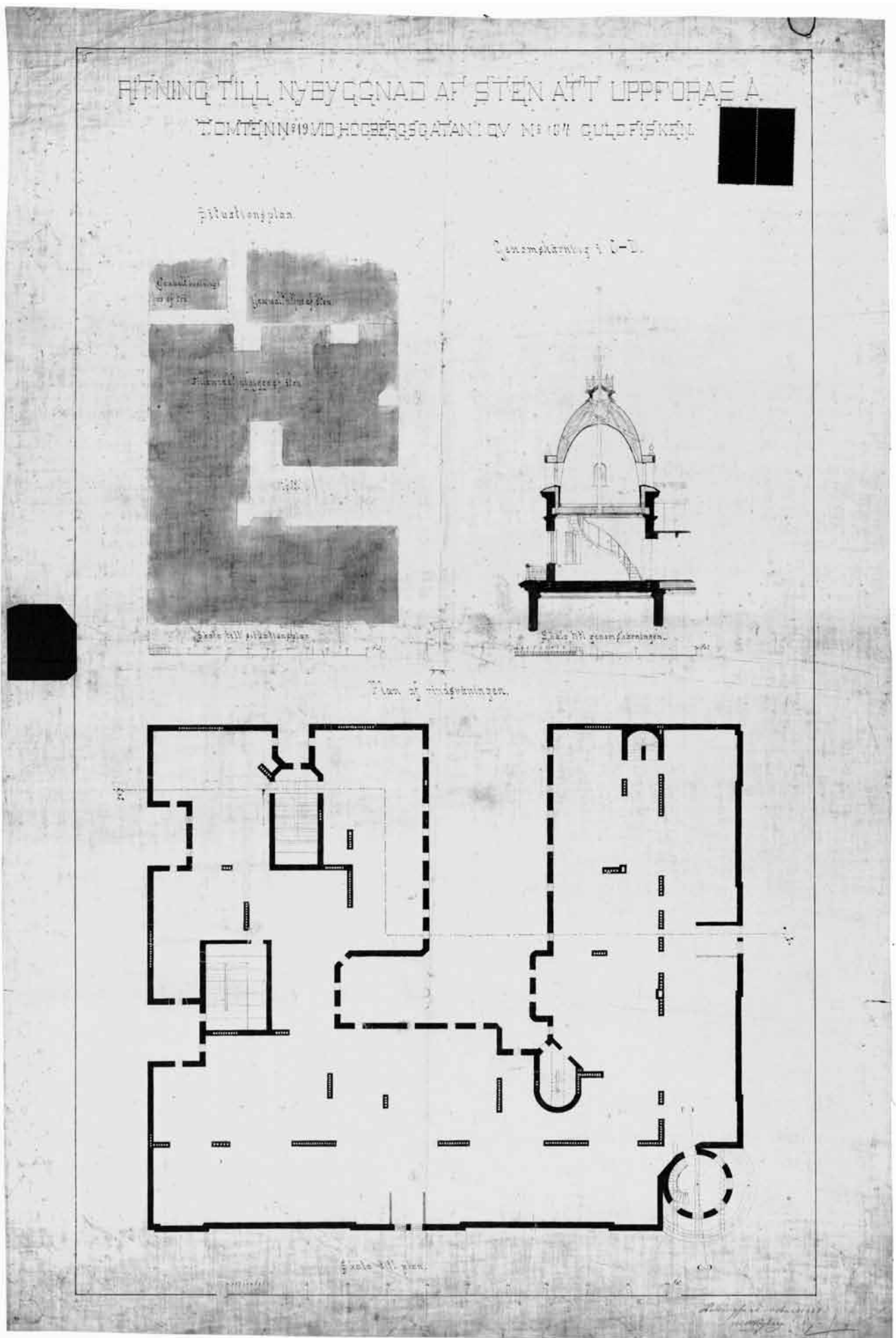
Asemapiirros, tornin yläosan leikkaus ja ullakkokerroksen pohja. Axel Höberg 1888. KA.
