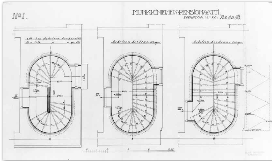
A-porrashuoneen työpiirustus n.1916.AM
