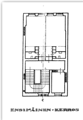
4. kerroksen eli ensimmäisen tornikerroksen pohjapiirros n.1916. RVV
