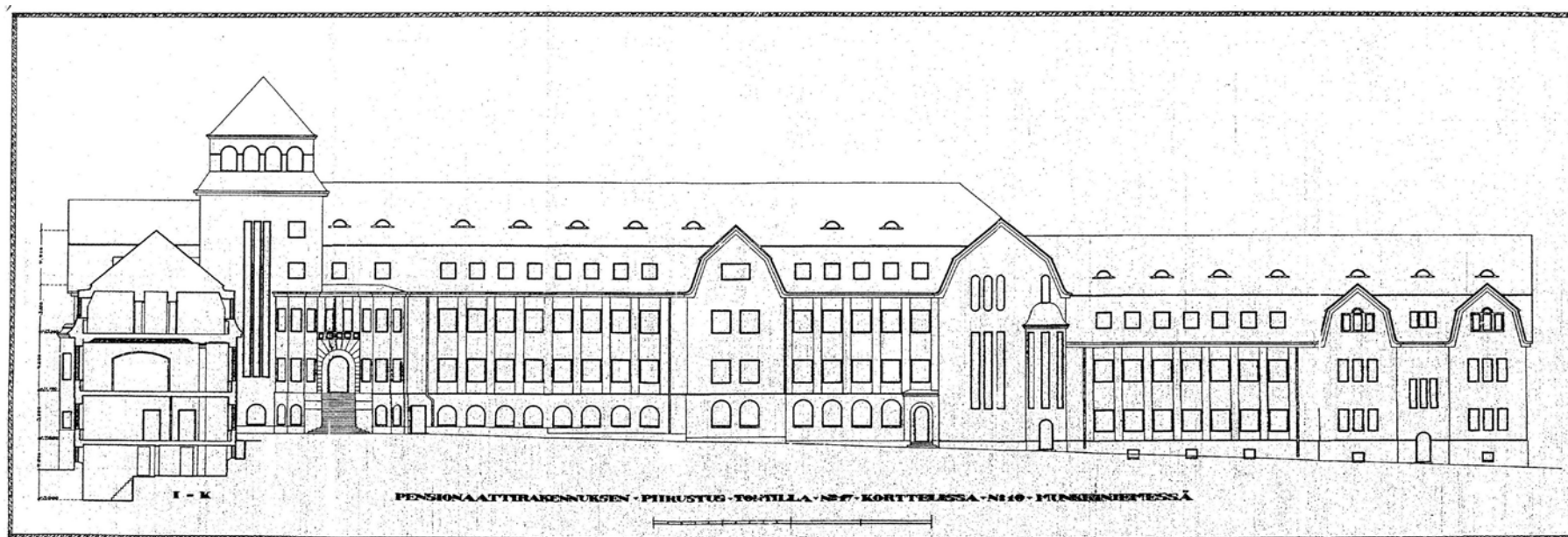
Munkkiniemen pensionaatin länsijulkisivun suunnitelma on päiväämätön, mutta luultavasti v.1916. RVV
