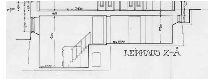
Osa leikkauspiirustuksesta n.1916, jossa vasemmalla pannuhuone (nyk.0011). Se muutettiin uima-altaaksi 1975 peruskorjauksessa.AM
