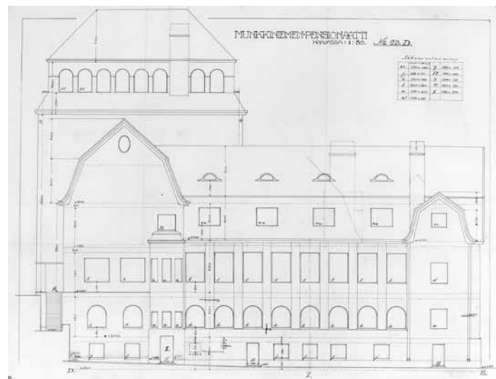
Pensionaatin pohjoisjulkisivun työpiirustus ikkunataulukkoineen n. v.1916.AM
