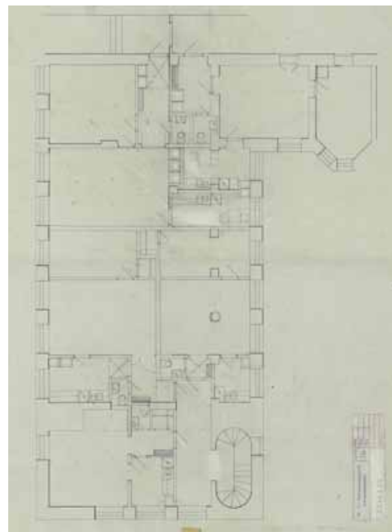
Suunnitelma keittiötilojen muutoksesta viideksi asunnoksi 1940- tai 50-luvulla. Puolustushallinnon rakennuslaitos
