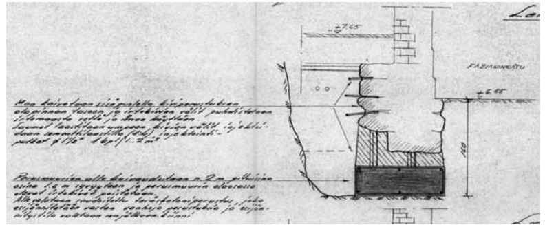
Vas: Arkkitehti E.B. Lohrmannin signeeraama pihasiiven leikkauspiirustus, jossa näkyy kantavat massiivitiiliseinät ja puurakenteiset välipohjat. KA
