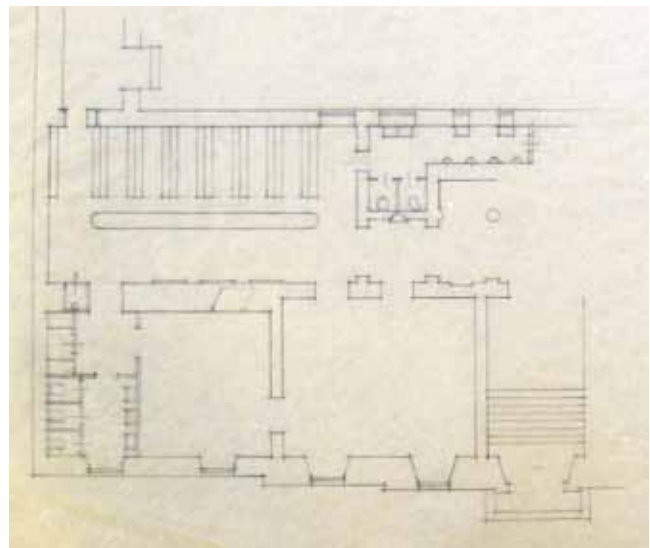
Rakennushallituksen arkkitehdin Gunnar Wahlroosin signeeraama luonnospöytäselitys 1. kerroksen itäpään muutoksista 28.6.1938, jossa näkyvät uudet vaatenaulakko- ja wc-tilat. KA
