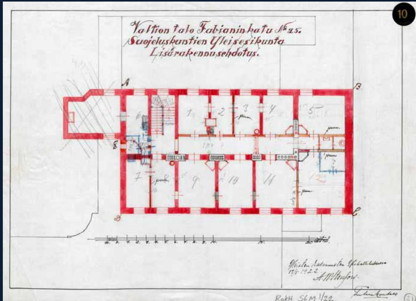
Pihasiiven korotuspiirustus 19.5.1922 (A. Stenfors / Yleisten rakennusten ylihallitus). KA
