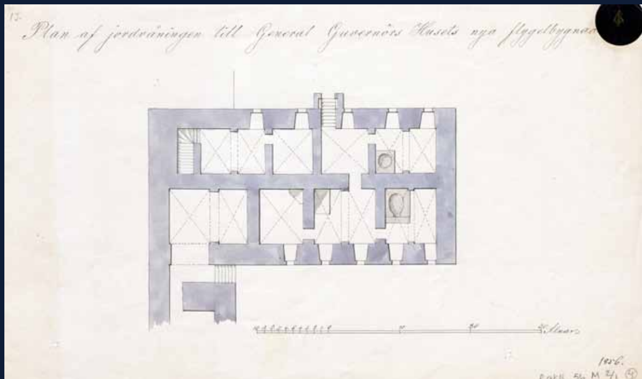
Pihasiiven kellarin pohjapiirros, johon on merkitty vuosiluku 1856. RakH / KA
