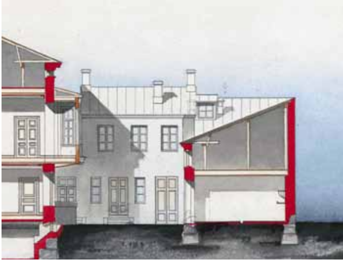
Ylinä itäsiiven julkisivut 1890-luvulta ja 1934. KA
