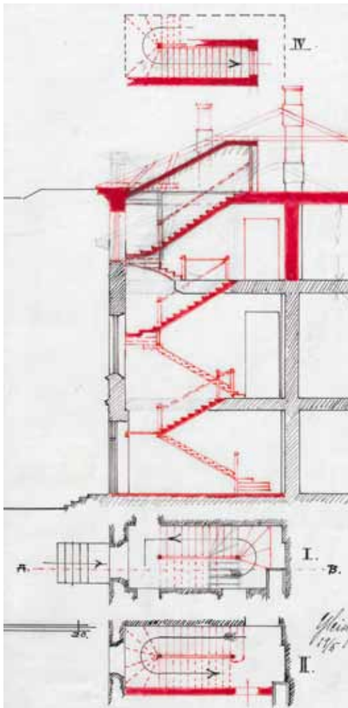
Osa pihasiiven korotuspiirustuksesta 19.5.1922 (Yleisten rakennusten ylihallitus / A. Stenfors), jossa on esitetty uusi porrashuone. KA
