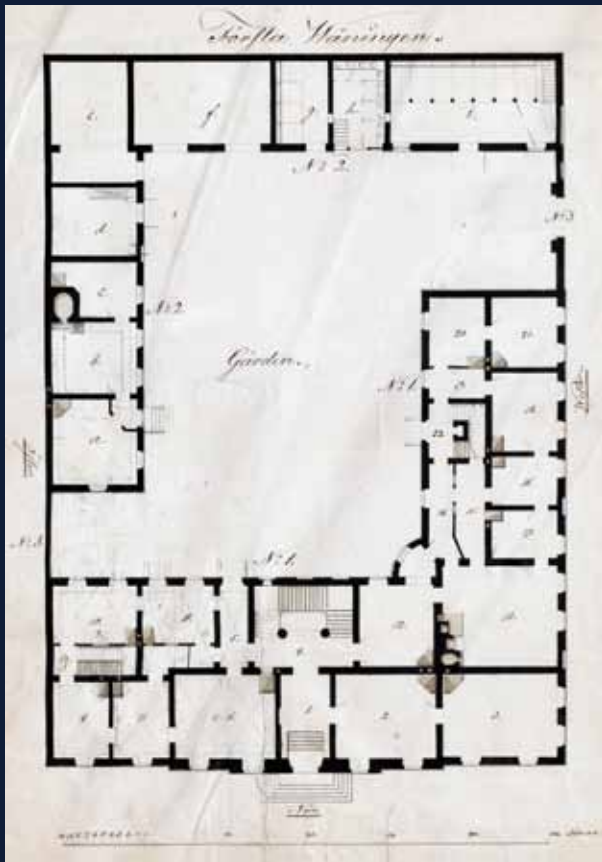
Ylitarkastajantalon ensimmäisen ja toisen kerroksen pohja- piirrokset 1820-luvun alusta. KA
