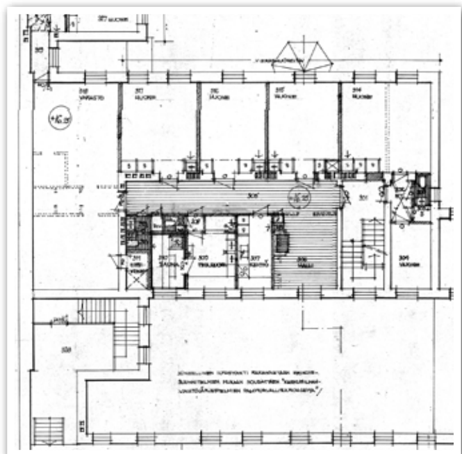
Pihasiiven kolmannen kerroksen muutokset 1960-luvun peruskorjauksessa. Osa pohjapiirustuksesta 11.7.1964 (Sirkka Tarumaa / Rakennushallitus). SKA
