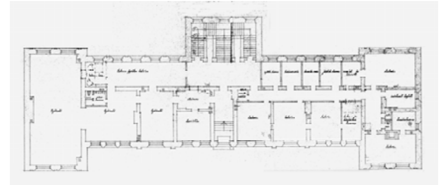
Sairaalan muutosluonnos - pohjakerrokseen laboratoriotiloja v. 1945 tai -46 VTT.
