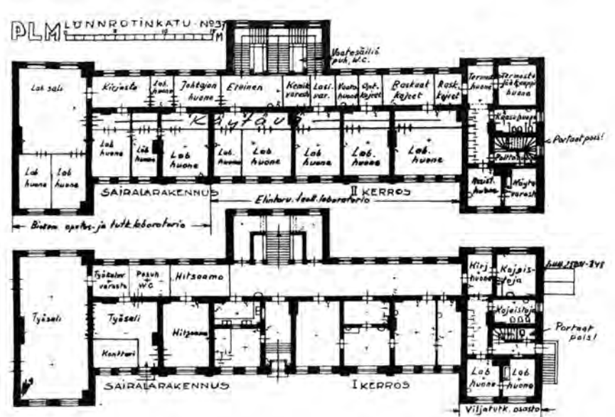
Tilakaavio vuodelta 1945, jossa näkyy VTT:n esittämä sairaalarakennuksen käyttöehdotus. Vanhat seinät ja säilyneet huonetilat erottuvat selvästi. KA
