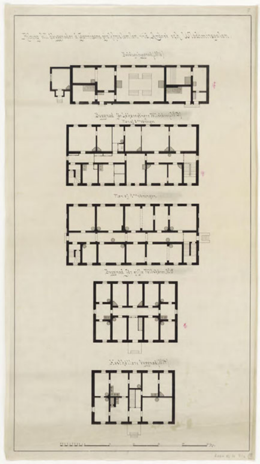
Sauna, vanha lasaretti, henkilökunnan asuinrakennus ja ruoanpitäjän rakennus, pohjapiirrokset 1880-l. KA
