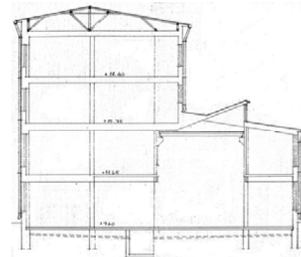
Jussi Paatelan luonnos vuodelta 1937 esittää Abrahaminkadun varrelle rakennettavaa rakennusteknillistä laboratoriotalota. Tuleva laajennus on esitetty Lönnrotinkadun puolelle. Lasaretin vanhat rakennukset olisivat joutunut väistymään hankkeen toteutuessa. Arkkitehti, liite 1937/ 10.
