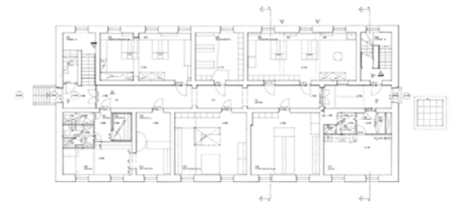
Vanhan lasaretin muutoslaboratorioksi. Pohjapiirroksat 1982. Arkk.tsto HLS. RVV, SKA
